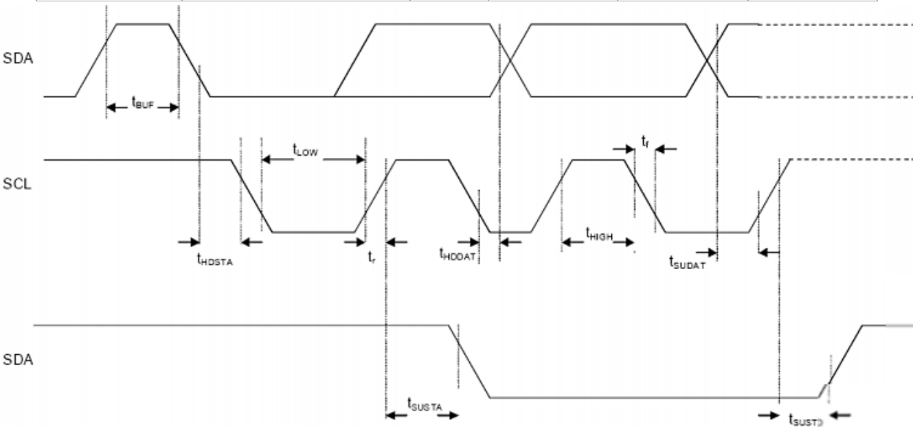
图 5. I2C 时序图
