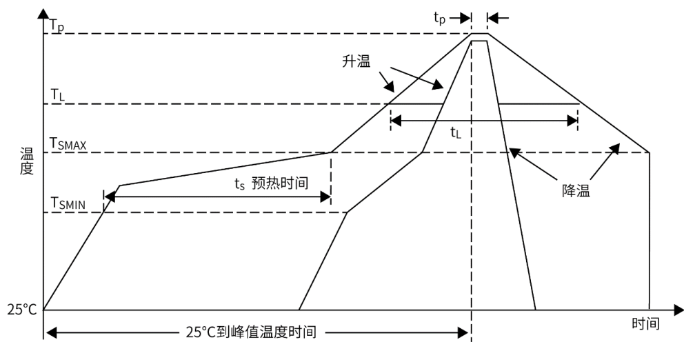
图 10. 推荐无铅焊锡回流温度曲线分布图
