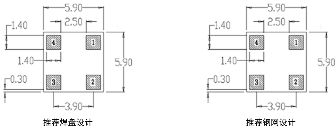
图 9. 推荐焊盘与钢网设计（单位：mm）
