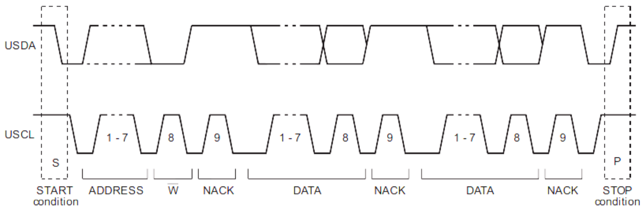
图 6. I2C 通讯协议
