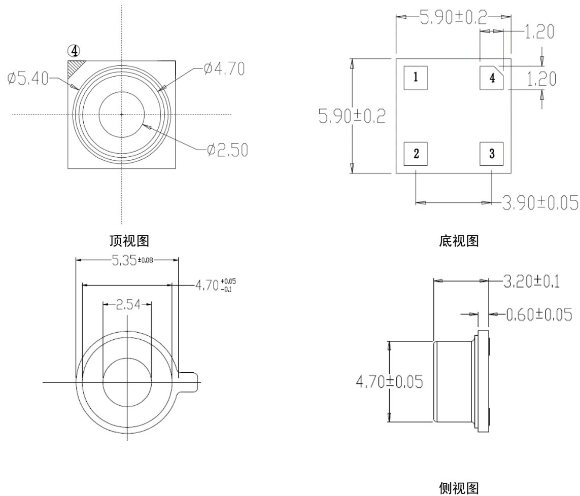
图 8.基底轮廓尺寸
