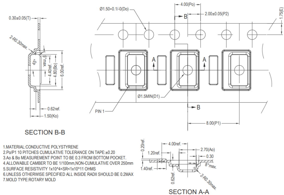
图 11-1 卷带尺寸
