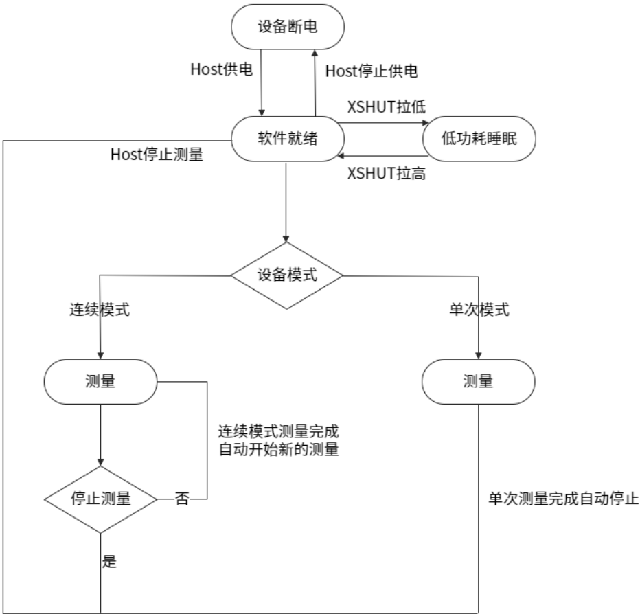
图 5-2 固件状态机
