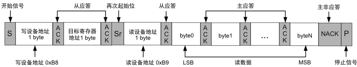
图 6-3 数据格式（读）
