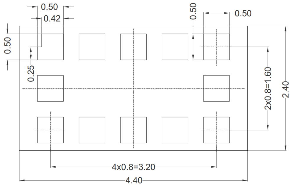
图 10-2 焊盘尺寸图 (Top View)
