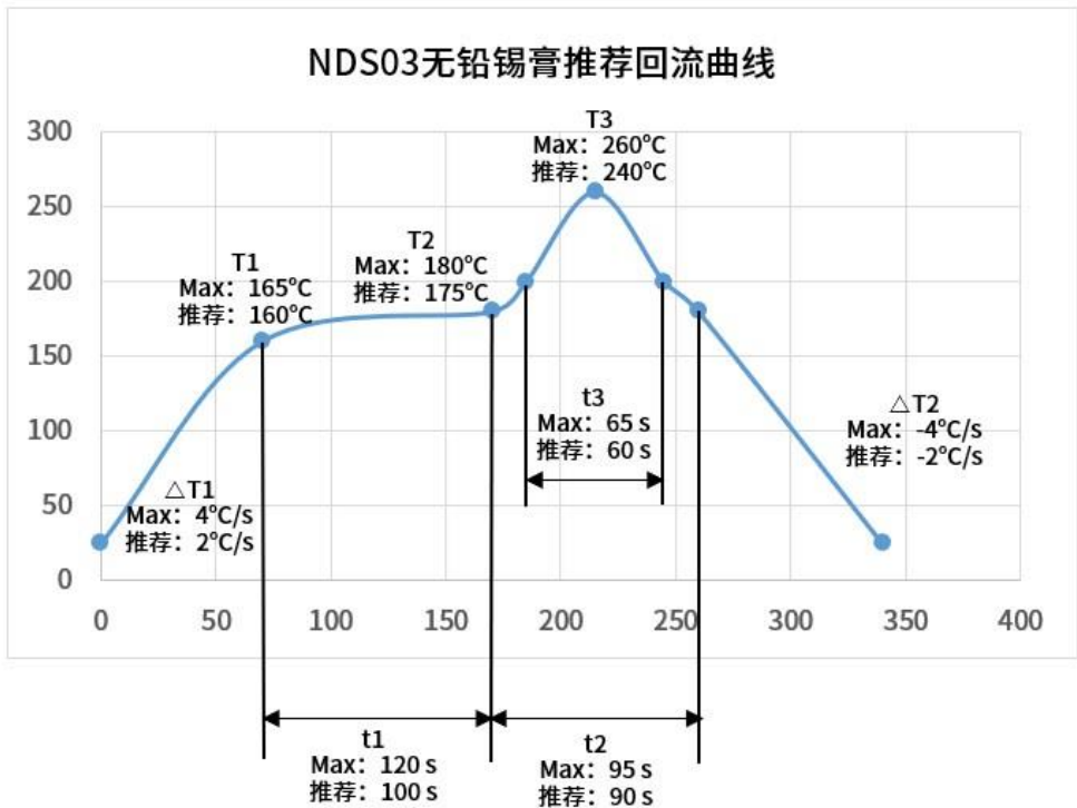
图 12-1 NDS03 无铅锡膏推荐回流曲线
