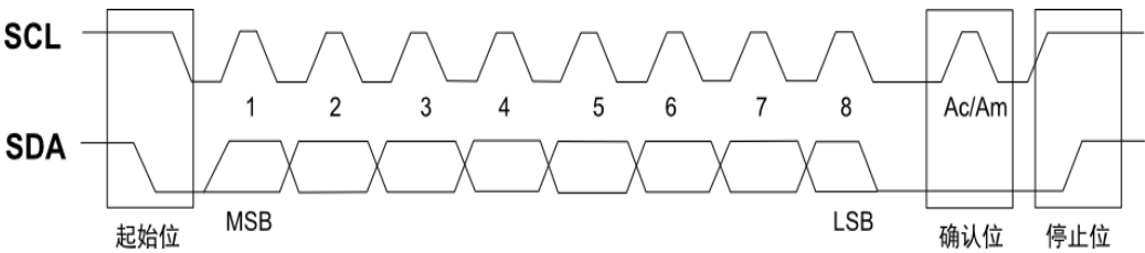
图 6-1 数据传输协议
