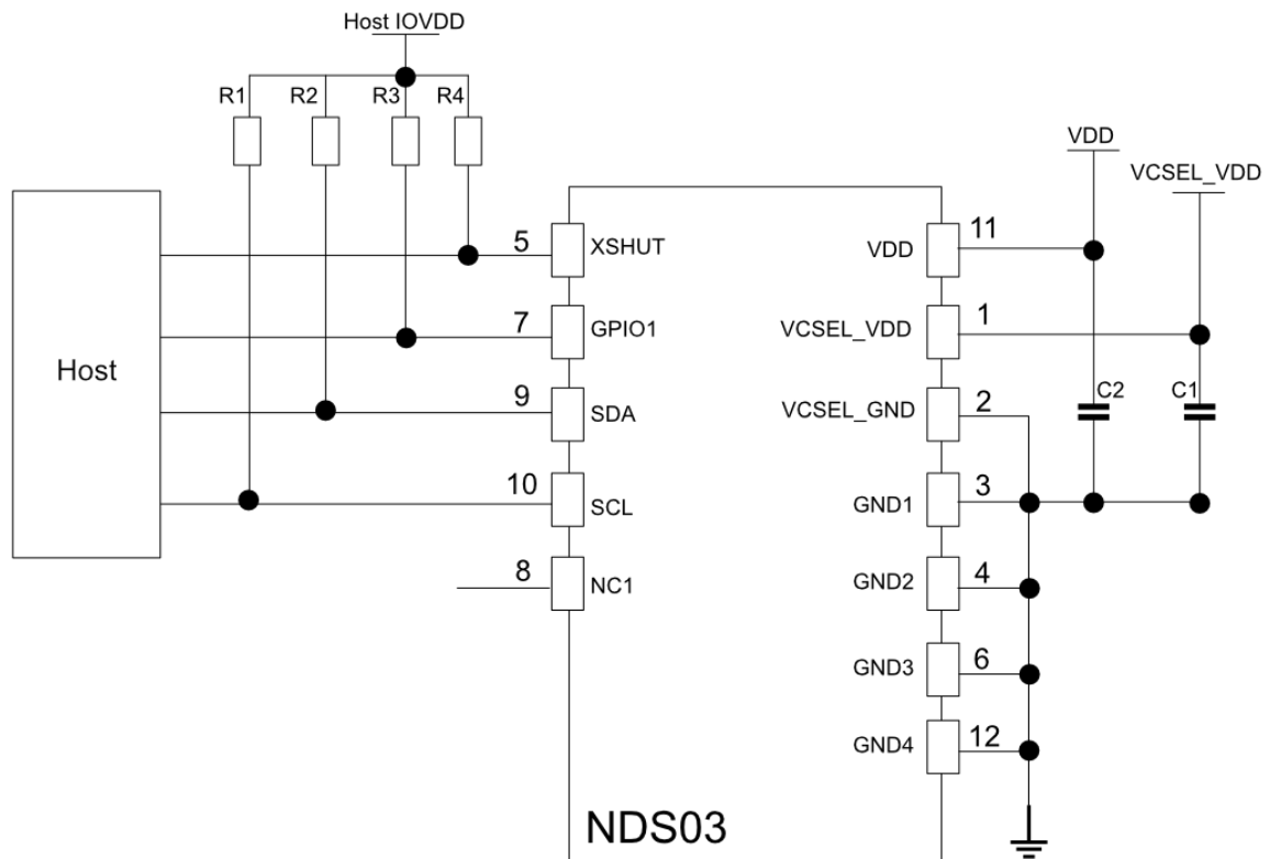
图 10-1 应用电路框图
