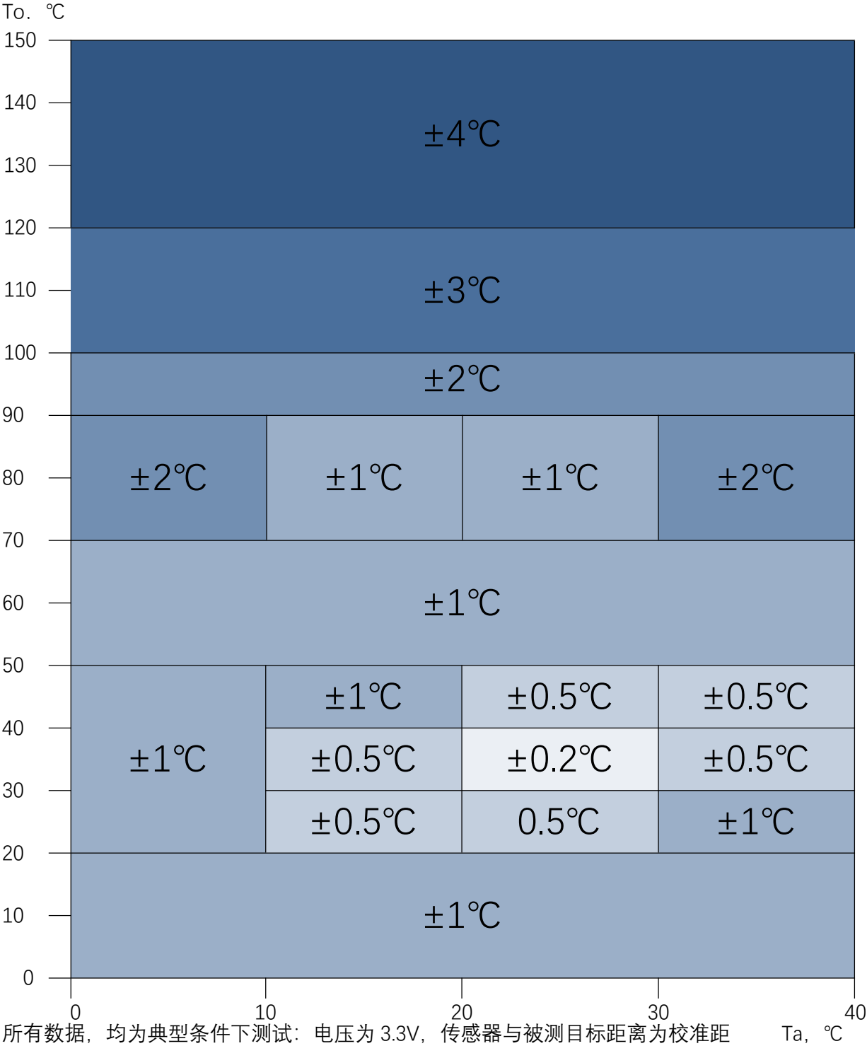
图 3 直插数字传感器 (Ta,To) 的标准精度
