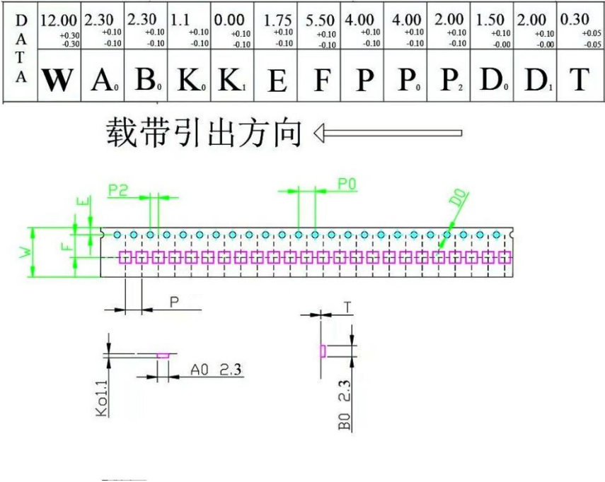
图 11 卷带式封装尺寸
