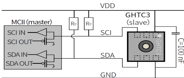
图 6 GXHTC3 的典型应用电路，包括上拉电阻和去耦电容 为了机械应力考虑，中心焊盘必须被焊接到地。
