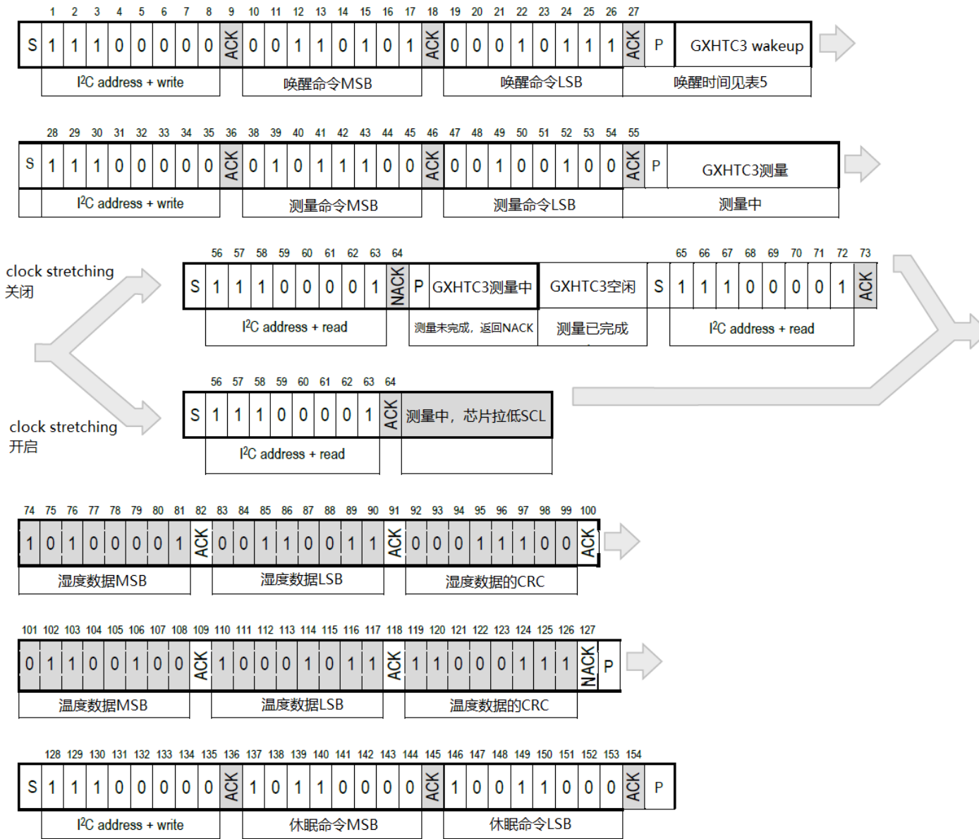
图 7 唤醒，开始温湿度测量，温湿度转换和休眠命令执行顺序示意图。 该示例展示的是湿度数据先发送，实际的湿度数据是 63%，温度 23.7° C，其中白色框是由微处理器控制，灰色框是由传感器控制。
