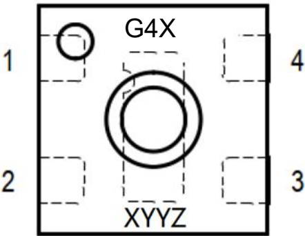
图 1 GXHT4x 顶视图
