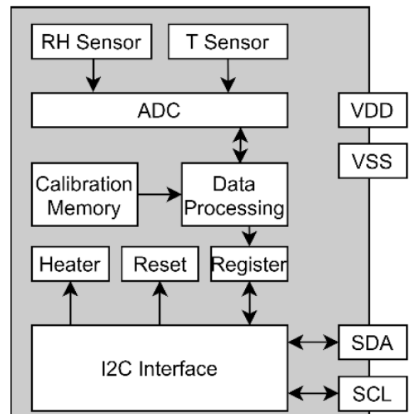
GXHT4x系列芯片功能框图
