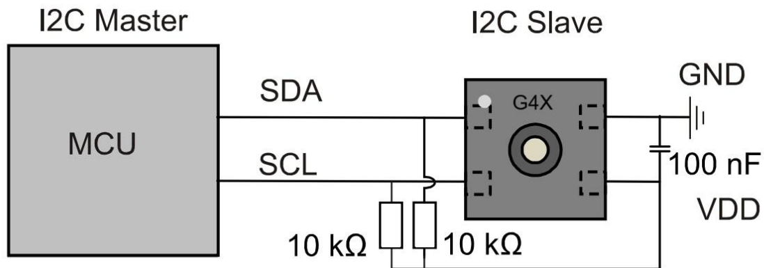
图 12 GXHT4x 典型应用电路参考图
