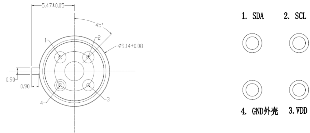
图 9 基体底视图
