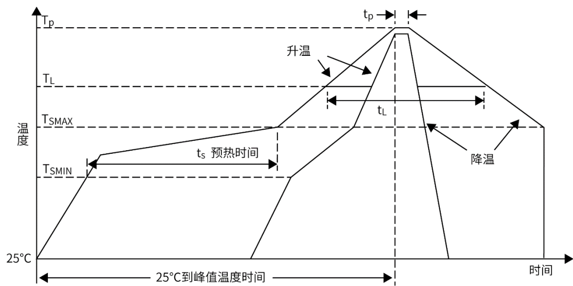
图 11 推荐无铅焊锡回流温度曲线分布图
