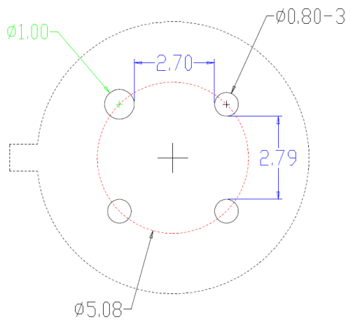
图 12 推荐焊盘设计
