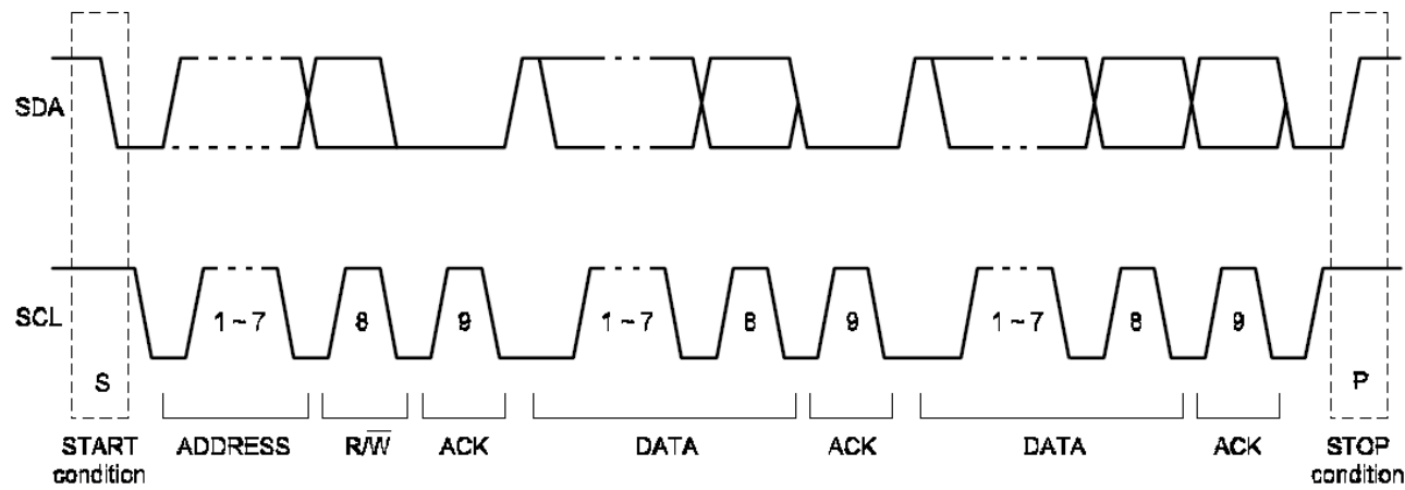
图 7 I 2 C 通讯协议
