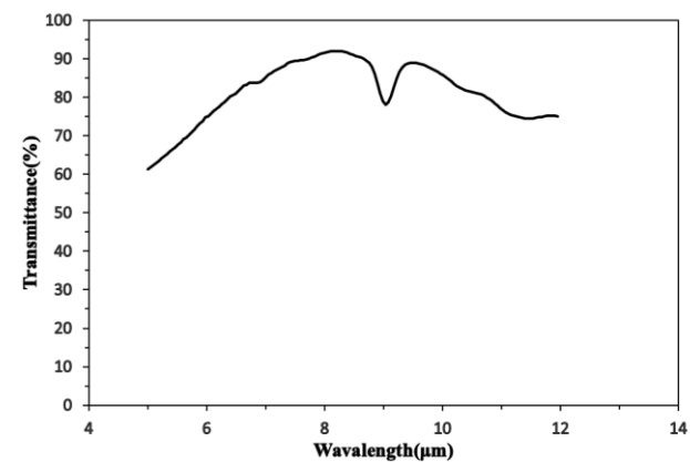
图 1 滤光片的透过光谱
