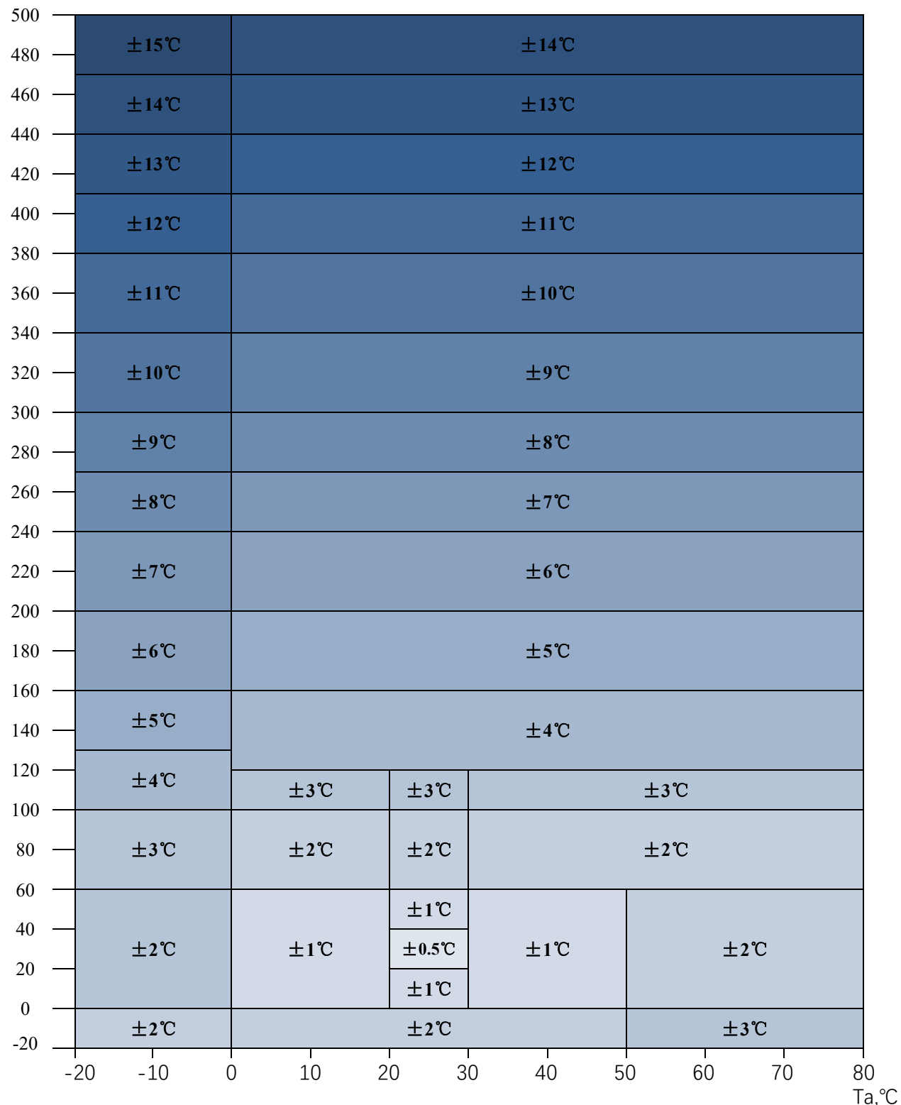
图 3 FW-TRS-5.5D3I (Ta, To) 的标准精度
