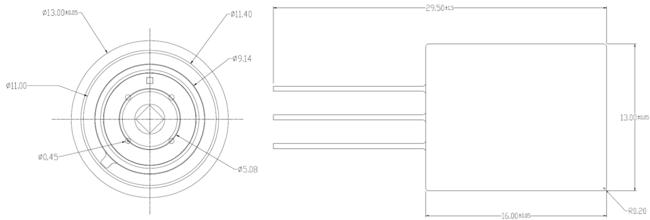
图 10 基体轮廓尺寸
