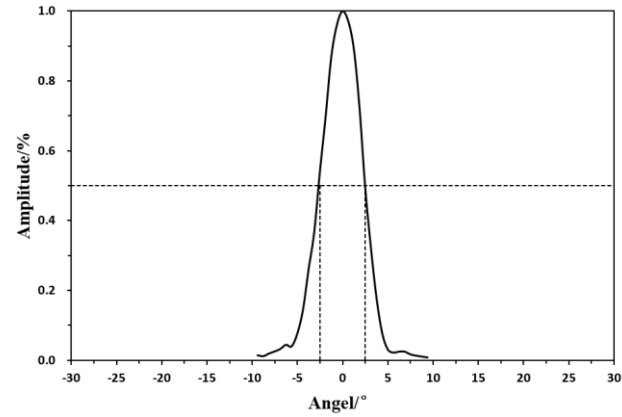
图 2 传感器的视场角
