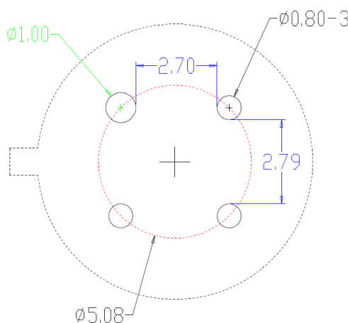
图 12. 推荐焊盘设计
