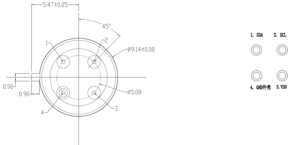
图 9 基体底视图
