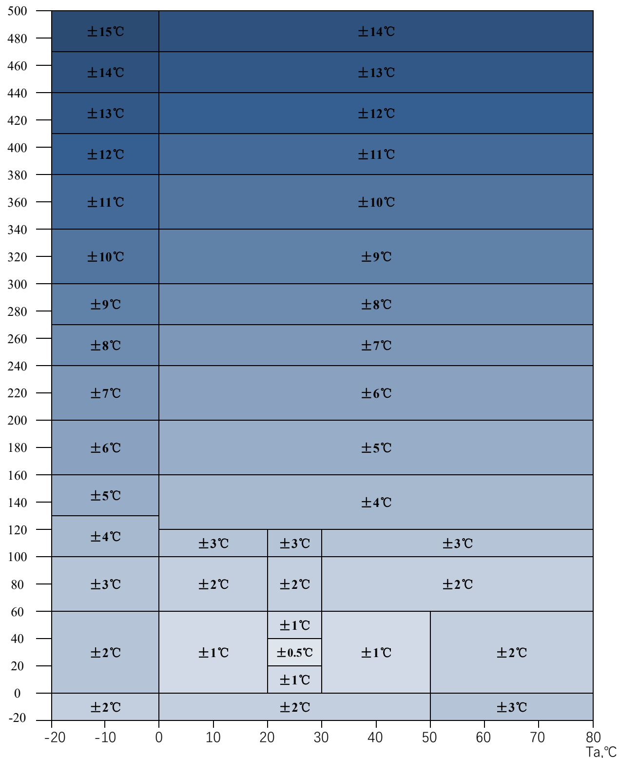
图 3. FW-TRS-5.5D1I/N1I ( T_a, T_o ) 的标准精度
