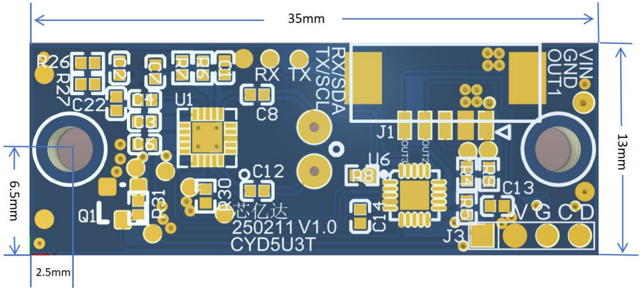
图 4.2 CYD5U3T 模块尺寸图
