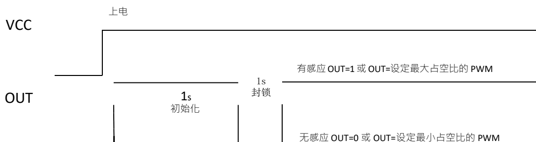
图 5.1 上电：OUT 引脚输出信号时序图
