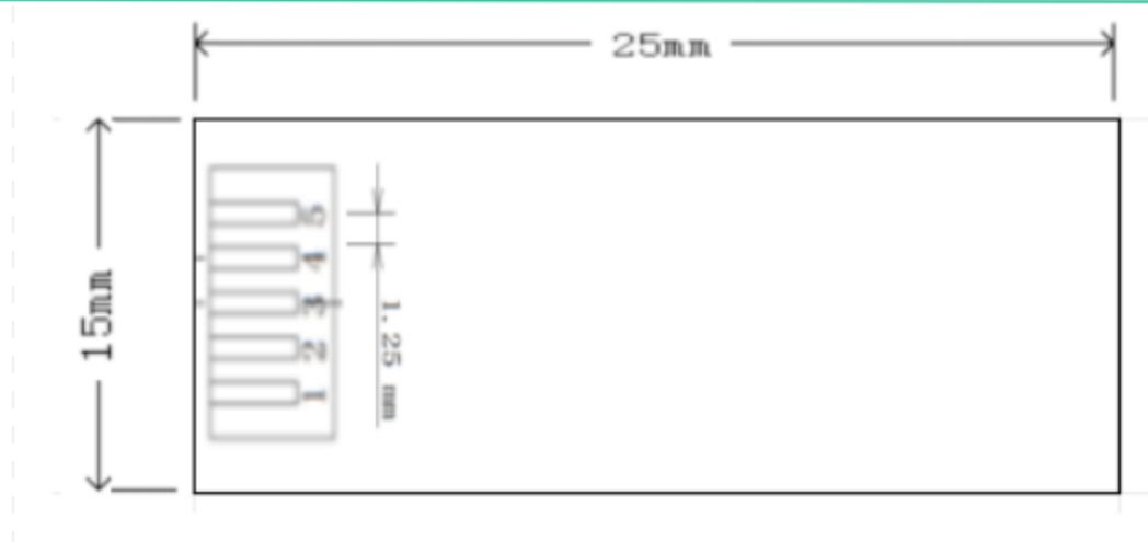
图 4.2 CYD58RD2515M 模块尺寸图
