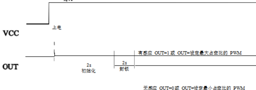
图 5.1 上电: OUT 引脚输出信号时序图
