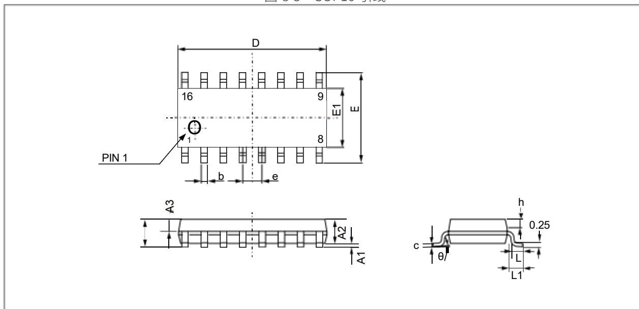
图 8-5 SOP16 引线
