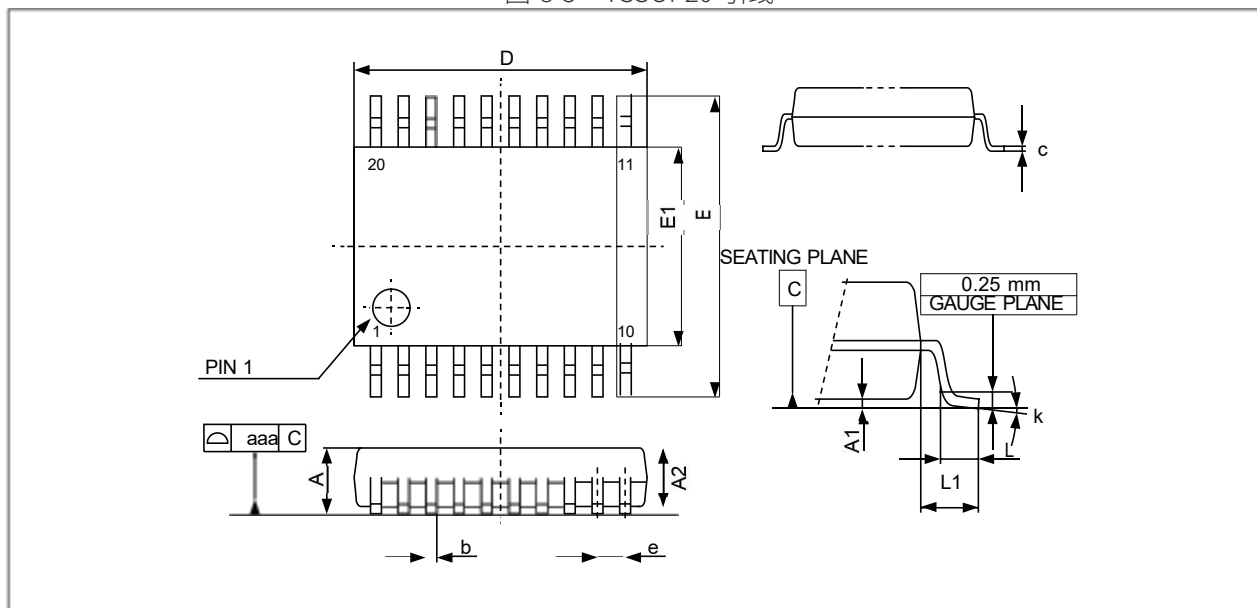
图 8-3 TSSOP20 引线
