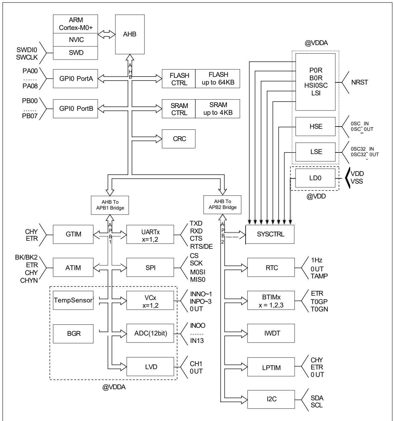
图 3-1 内部框图
