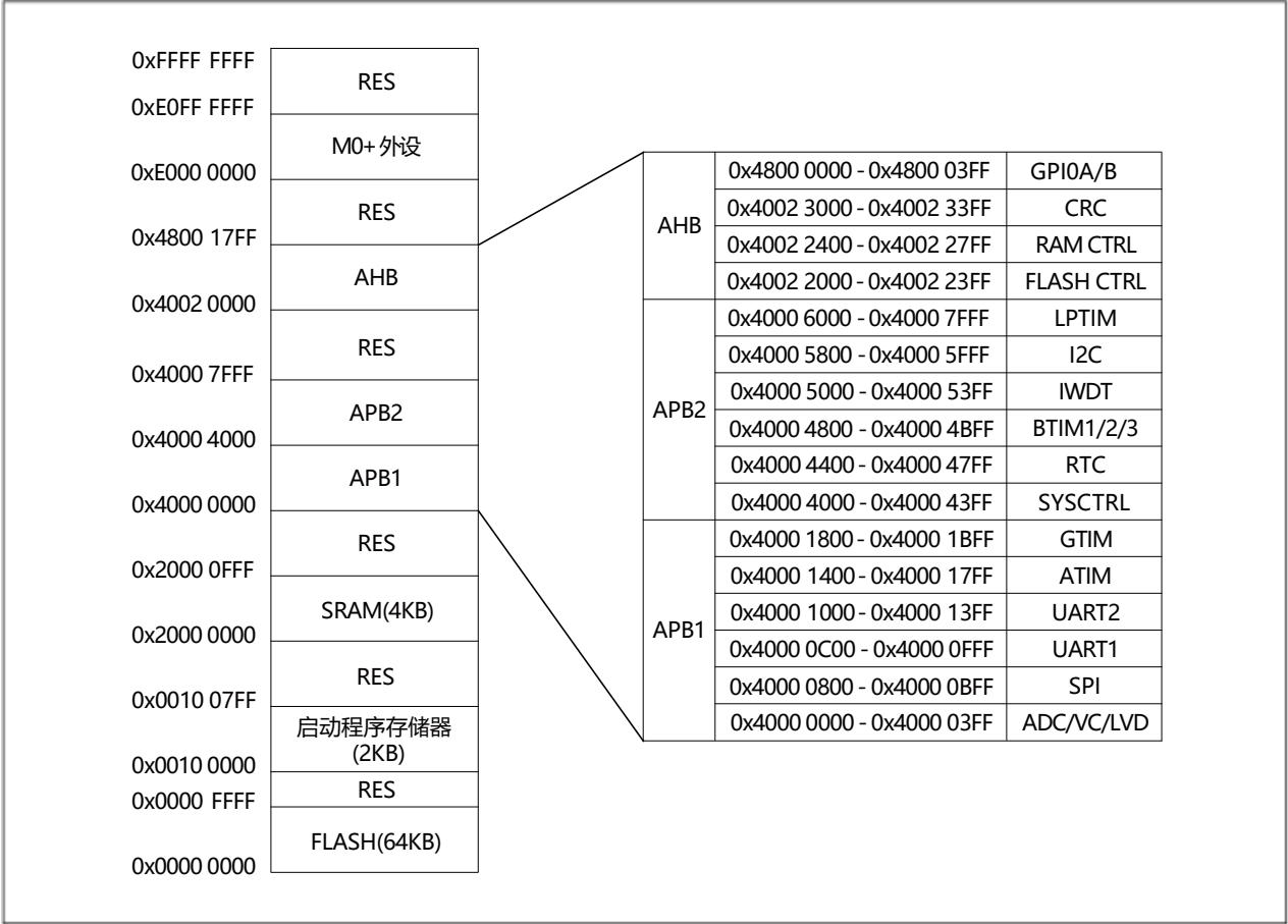
图 6-1 CYD010 的内部地址镜像
