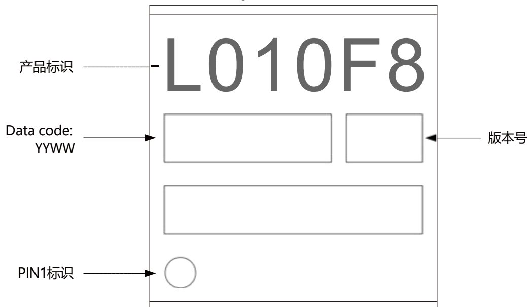
图 8-2 QFN20 顶部标记示例
