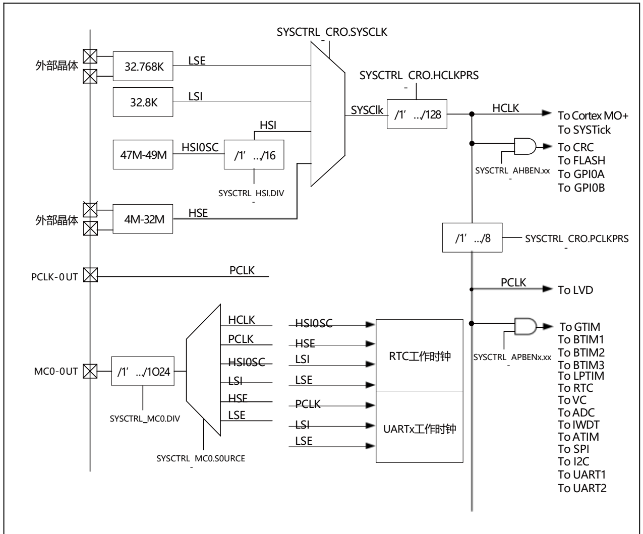
图 4-1 CYD010 的时钟树
