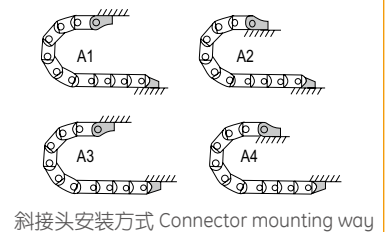
斜接头安装方式 Connector mounting way
