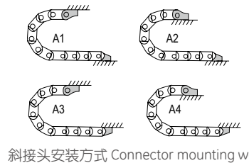
斜接头安装方式 Connector mounting way
