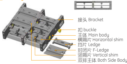
示意图 Drawing
