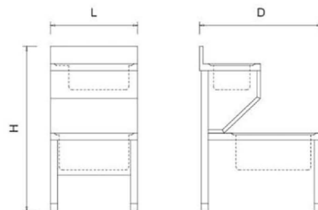
高低拖把池 / High And Low Mop Pool
