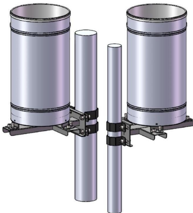
立杆直径为48mm/76mm，用两个抱箍固定
