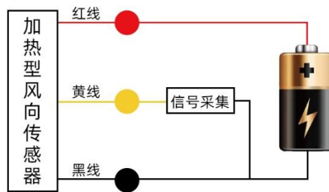
(电压、4~20mA单路供电)
