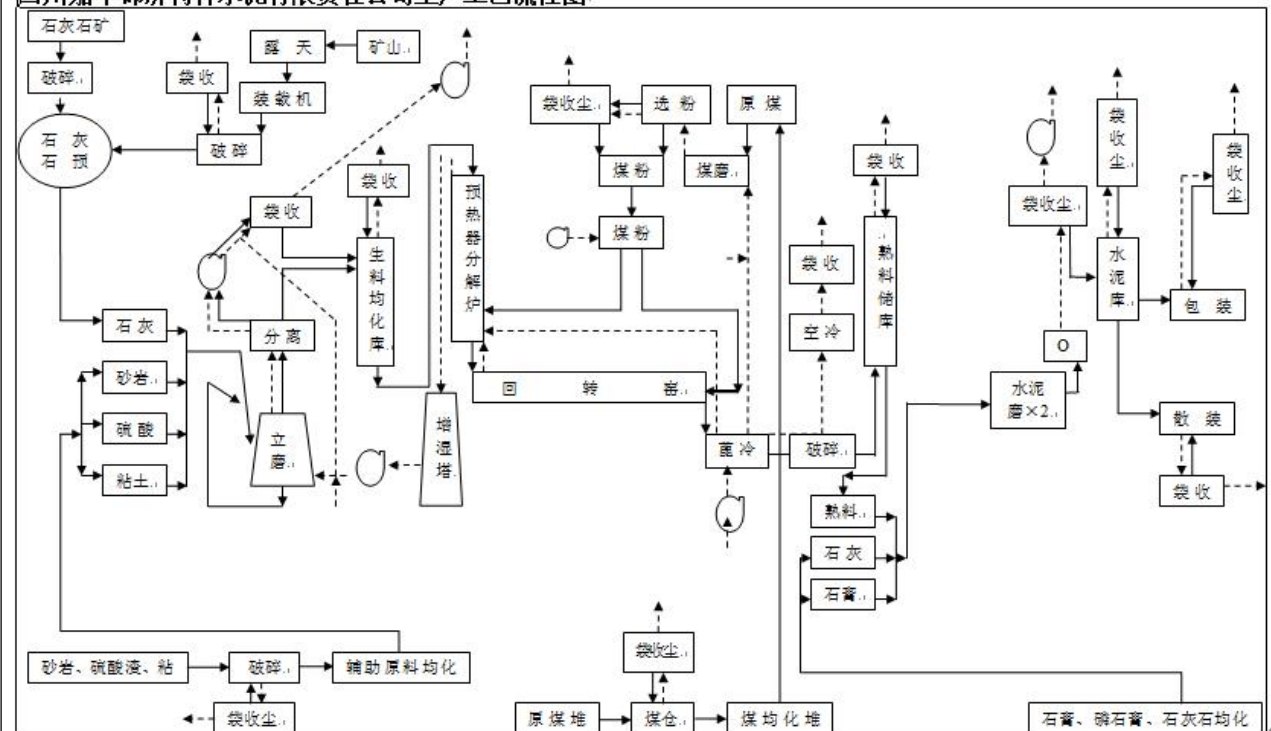
图 2 工艺流程图
