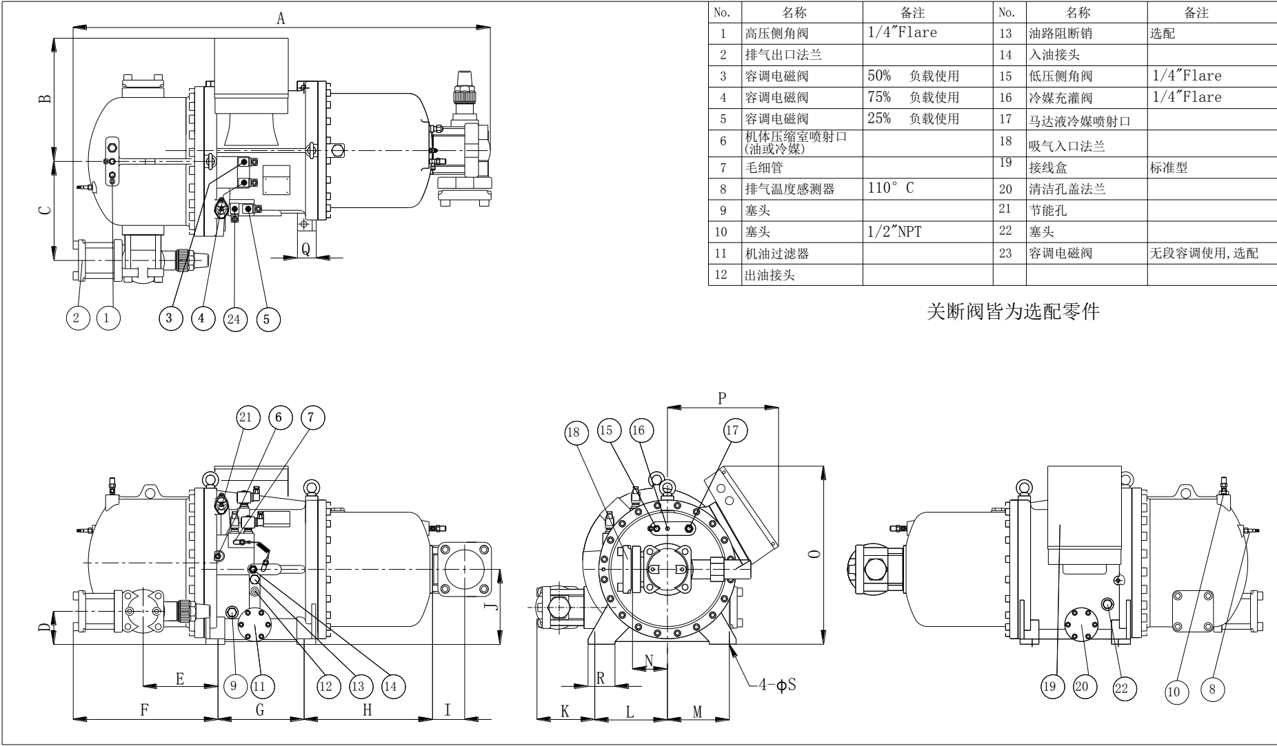
RC2 -200A&B~620A&B (RC2 -620A&B 水平吸气口) 外观图(水平排气)
