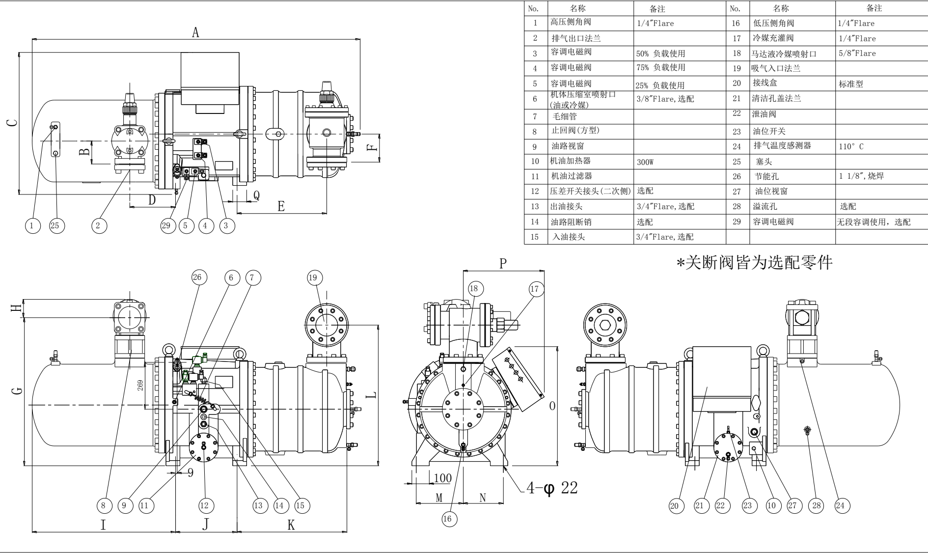
RC2 -620A&B~930A&B（RC2 -620 垂直吸气口）外观尺寸图
