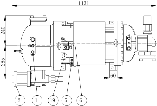
RC2 -180A& B-P 外观图(水平排气)
