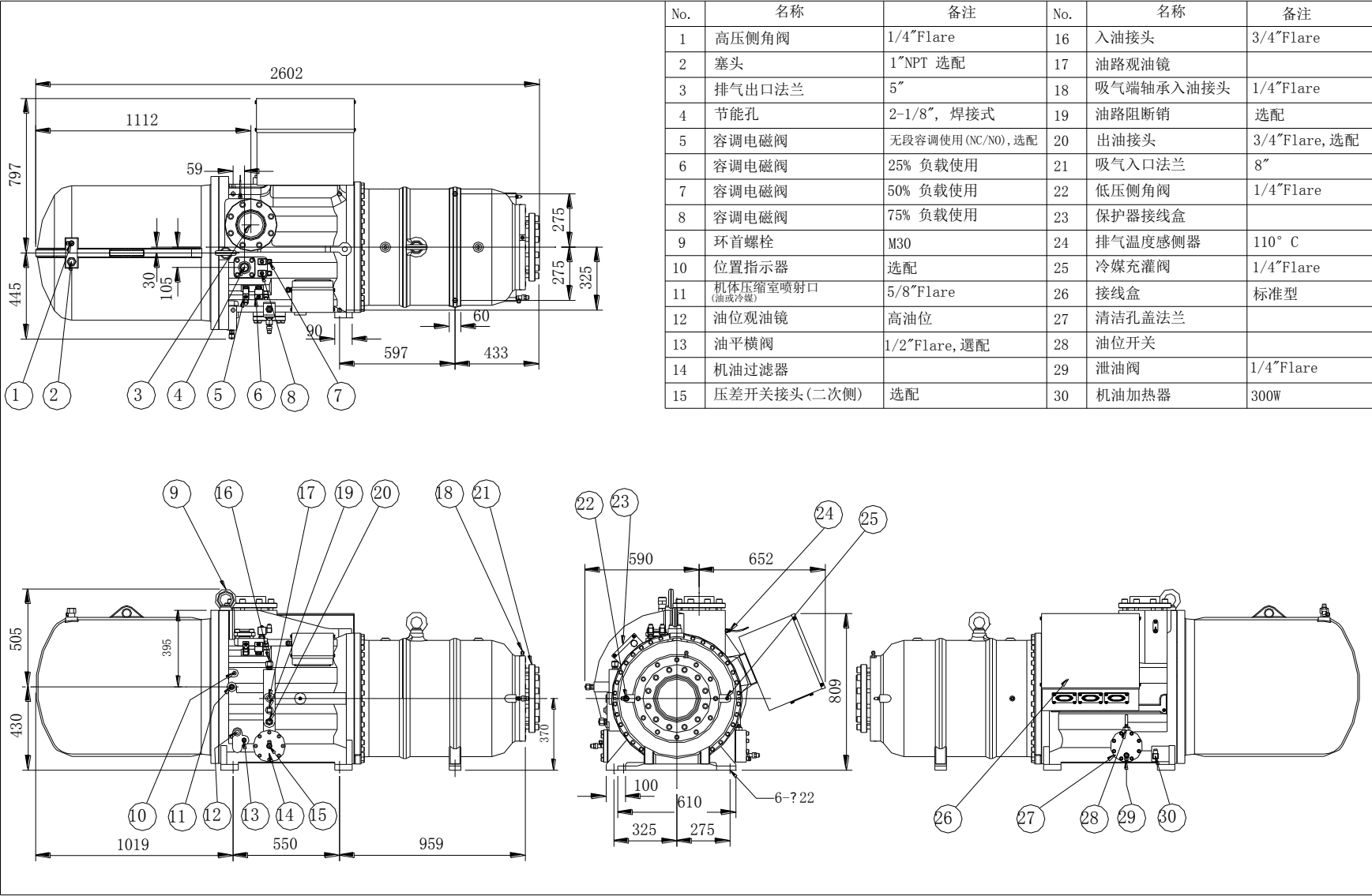
RC2 -1270/1530A&B HV 高电压外观图
