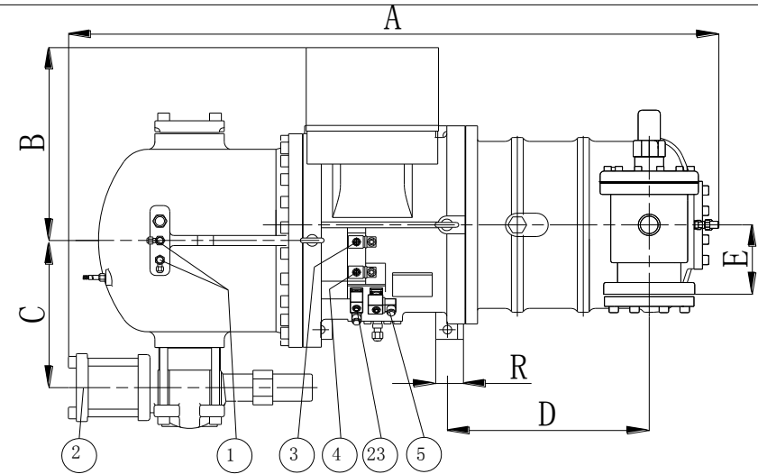
RC2 -620 A&B~930 A&B-P 垂直吸气口外观图(水平排气)
