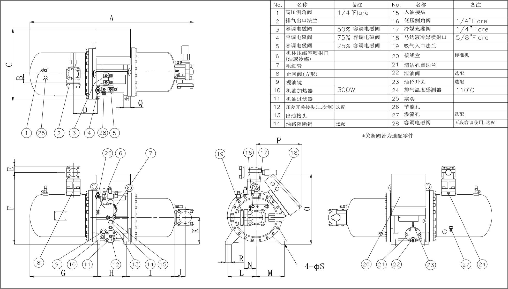
RC2 -200A&B~620A&B (RC2 -620 水平吸气口) 外观尺寸图
