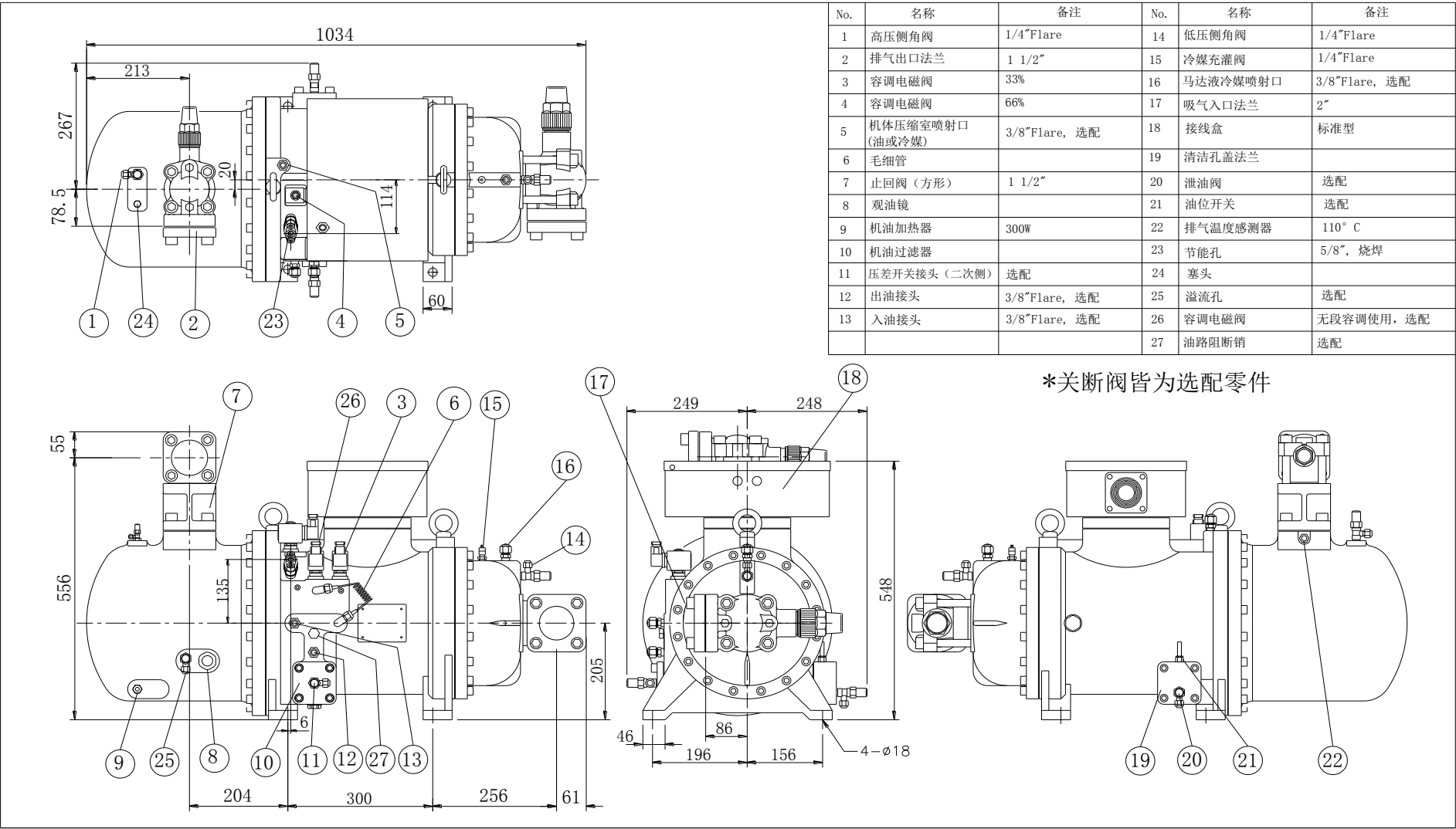
RC2 -100~RC2 -140 A&B 外观尺寸图
