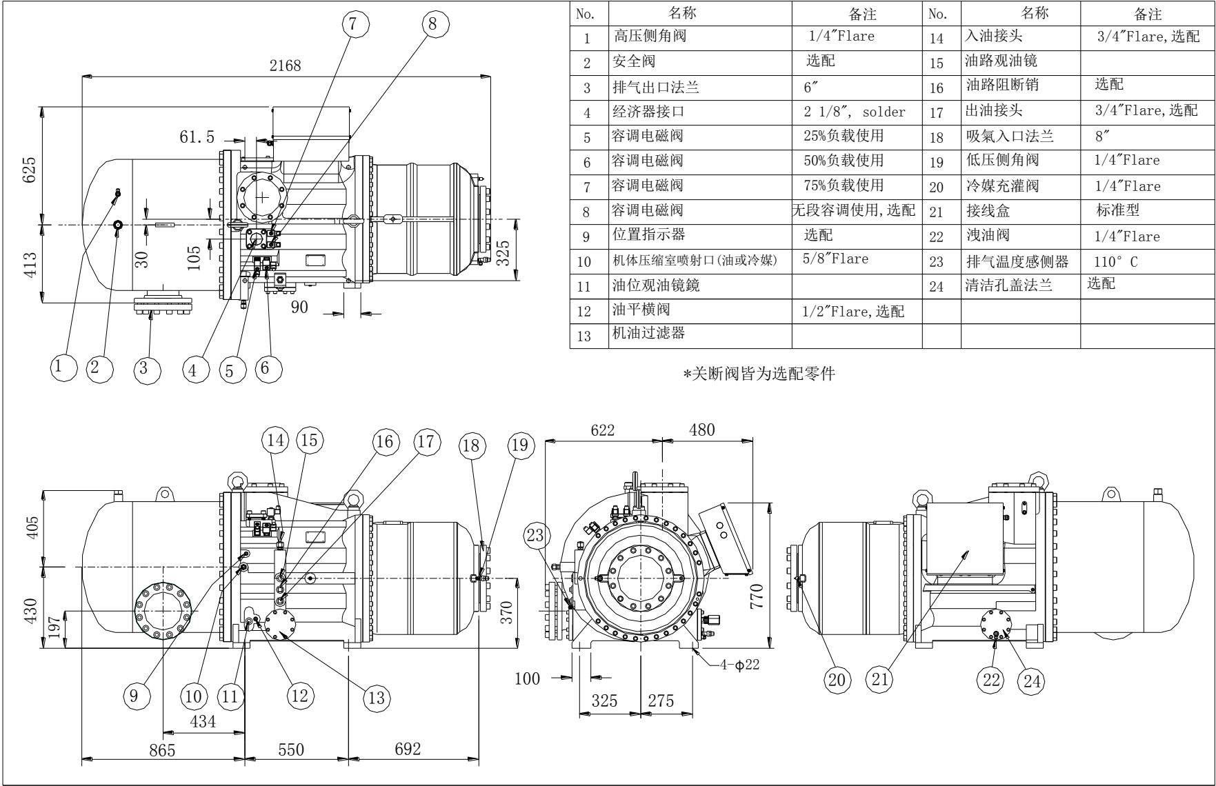
RC2 -1270/1530 外观图(水平排气)
