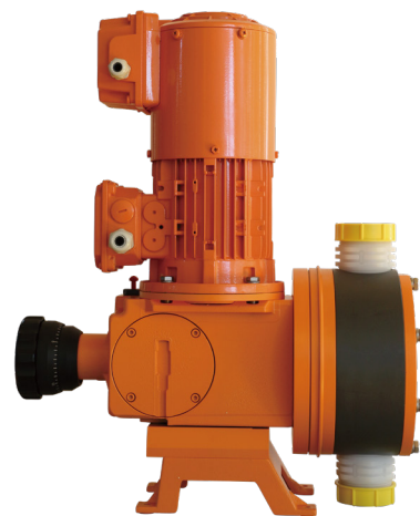
型号：Meta S电机驱动计量泵 流量范围：1030 l/h
