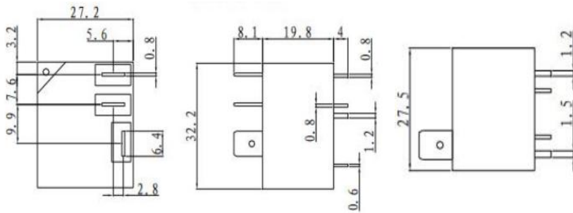
外形尺寸 Outline Dimensions
