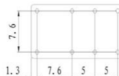
安装孔位图(底视图) Installation hole bitmap
