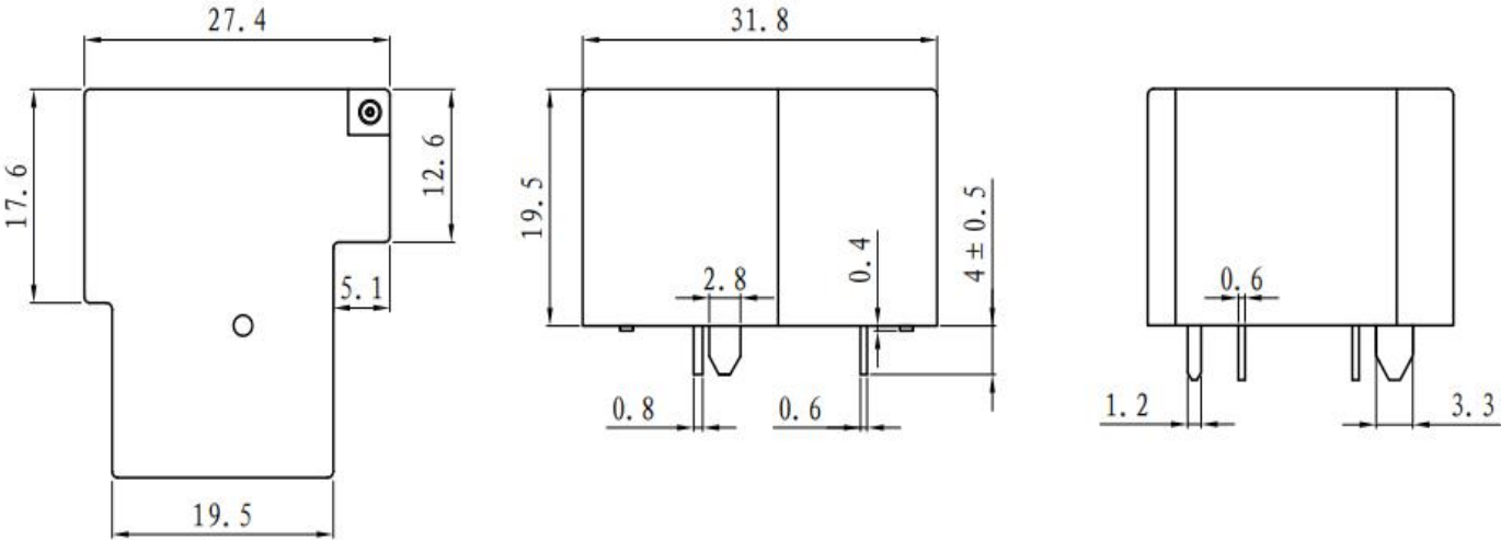
外形尺寸 Outline Dimensions
