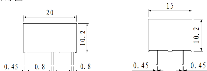
外形图
