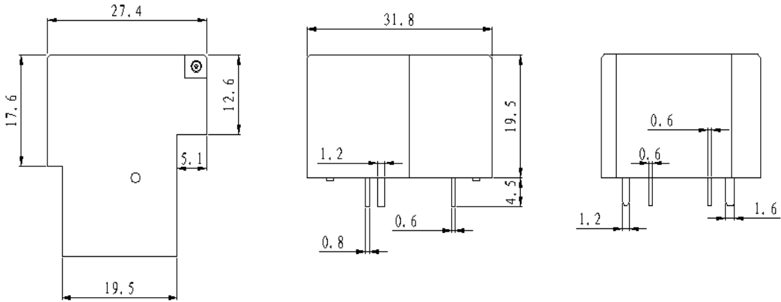
外形图
