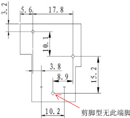
安装孔位图（底视图）
