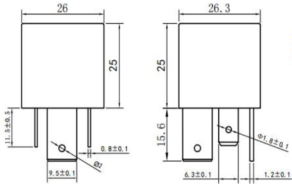
外形图 Outline Dimensions
