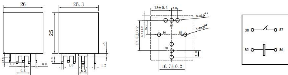
接线图（底视图） Wiring Diagram (Bottom View)
