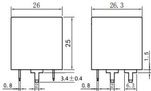
外形图 Outline Dimensions
