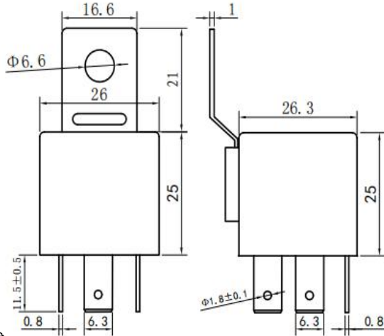
PCB板式 PCB board type
