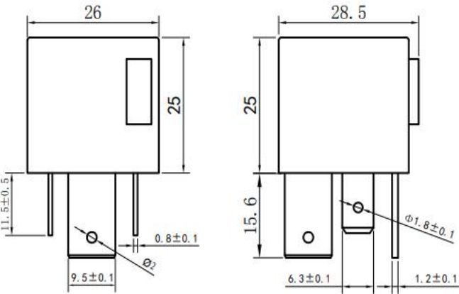
外形图 Outline Dimensions
