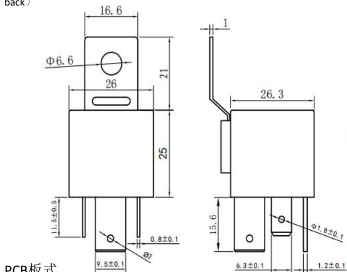
PCB板式 PCB board type
