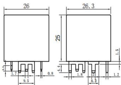
外形图 Outline Dimensions
