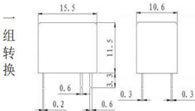
外形尺寸 Outline Dimensions
