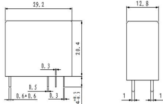
外形尺寸Outline Dimensions
