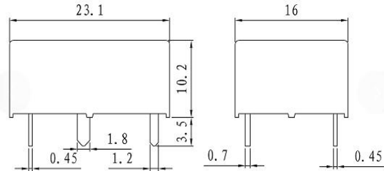
外形尺寸 Outline Dimensions
