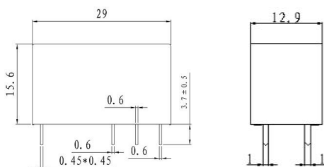
外形尺寸 Outline Dimensions
