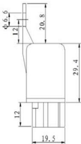
外形尺寸 Outline Dimensions
