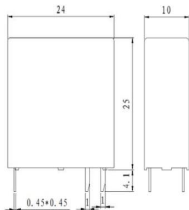
外形尺寸 Outline Dimensions
