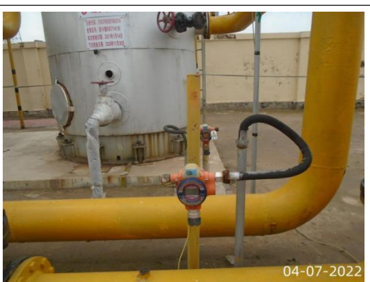
固定式硫化氢报警器
