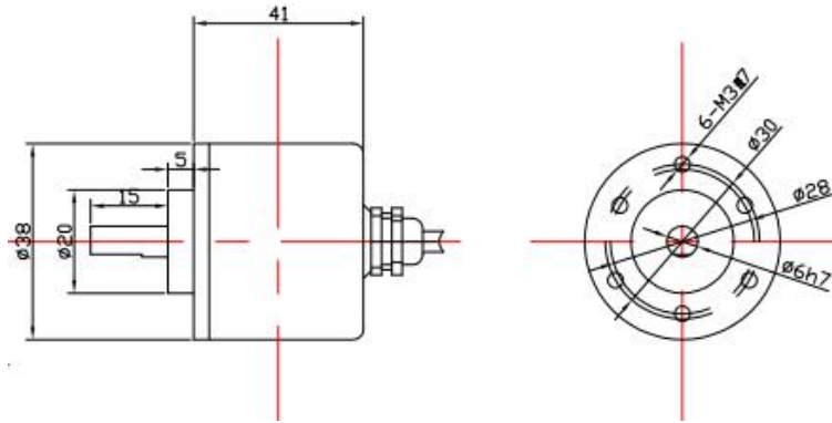
38mm 外径 6mm 轴径可选 15mm 轴长 径向出线可选
