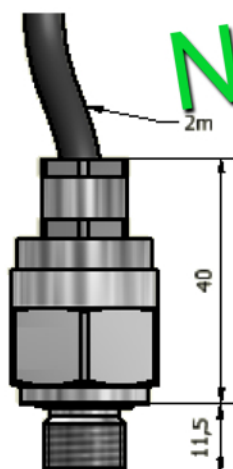
TR2/C2
