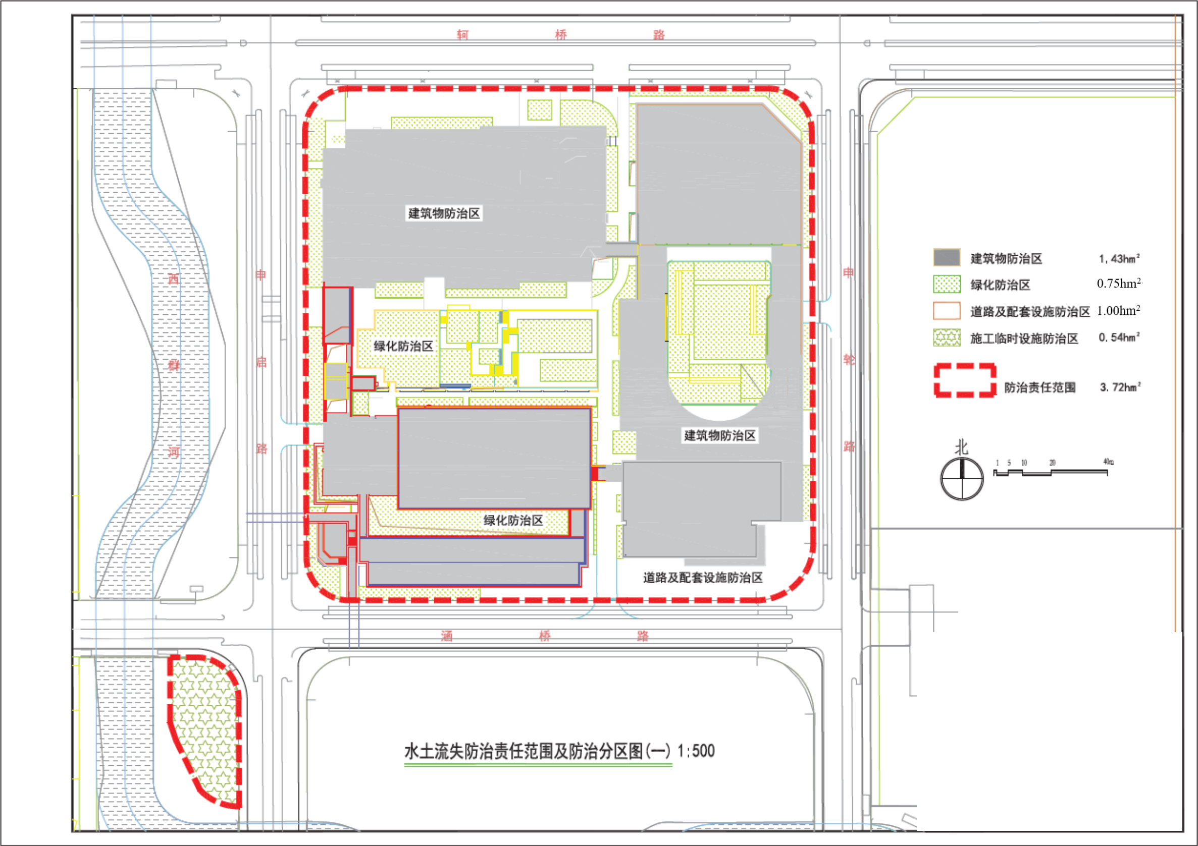
附图 2 金鼎天地培训中心项目分区防治措施总体布局图
