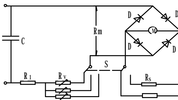
d) 测量泄漏电流装置的电路图
