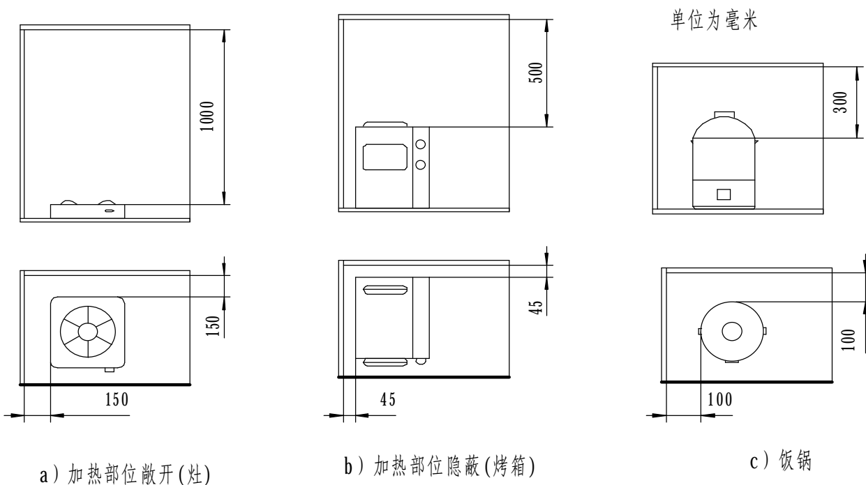
图 9 木壁、木台表面温升试验装置
