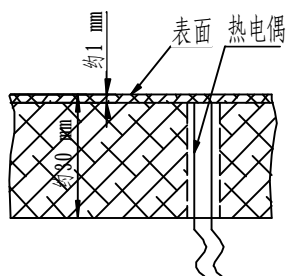
a) 埋热电偶
