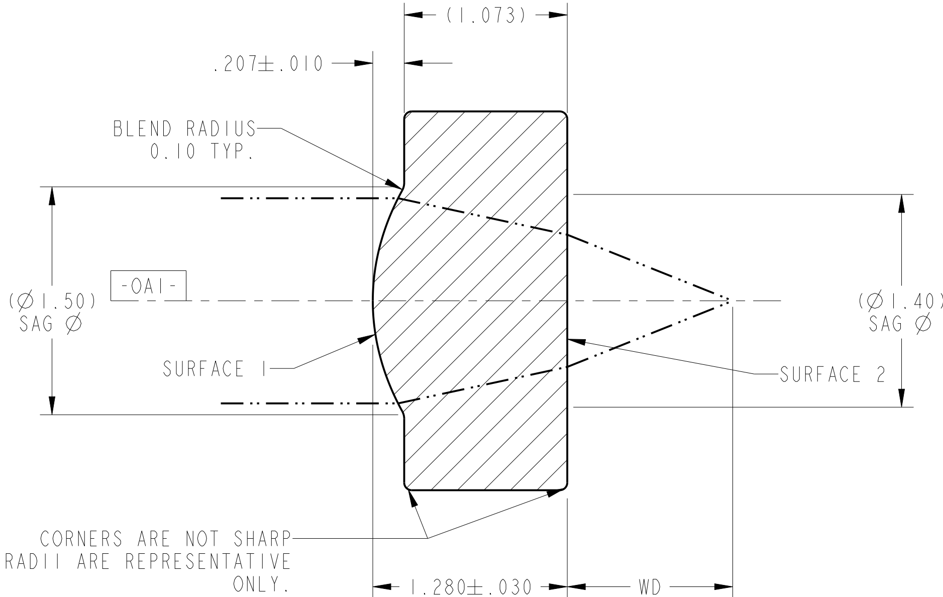
SECTION A-A
