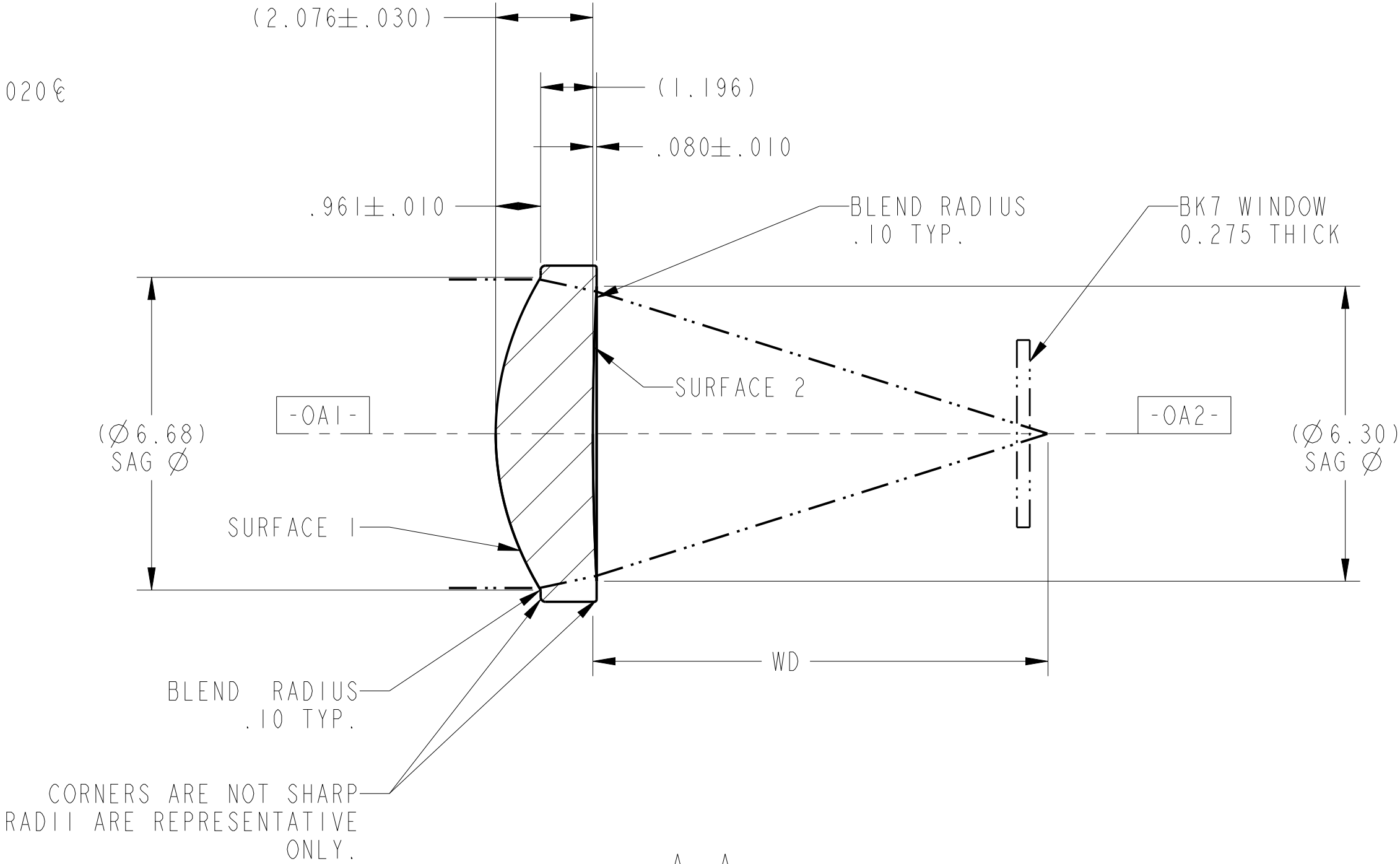
SECTION A-A
