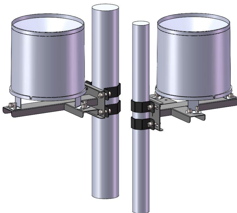
立杆直径为48mm/76mm，用两个抱箍固定
