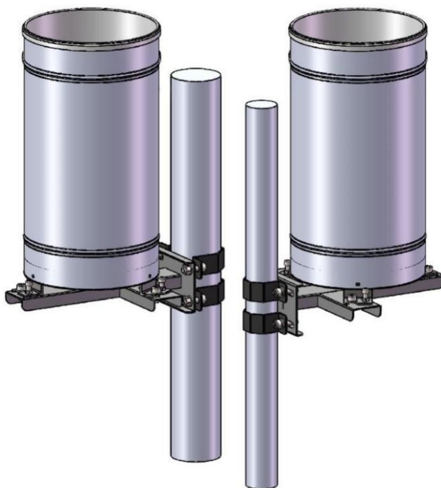
立杆直径为48mm/76mm，用两个抱箍固定
