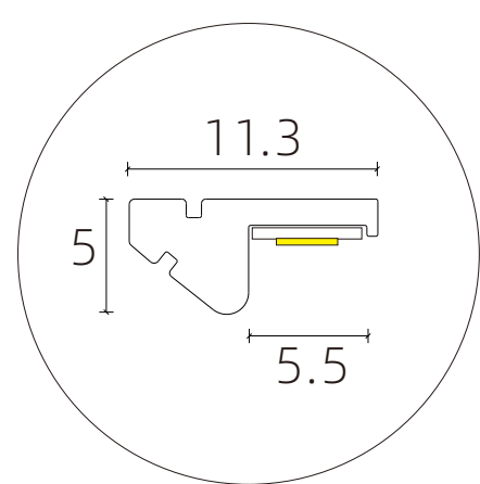
灯带铝型材
