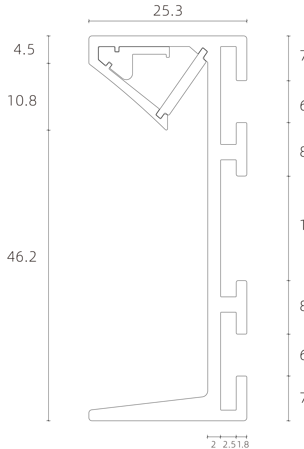
D6225铝型材
