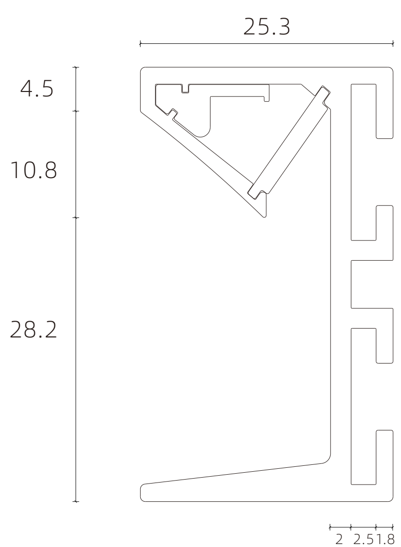
D4325铝型材
