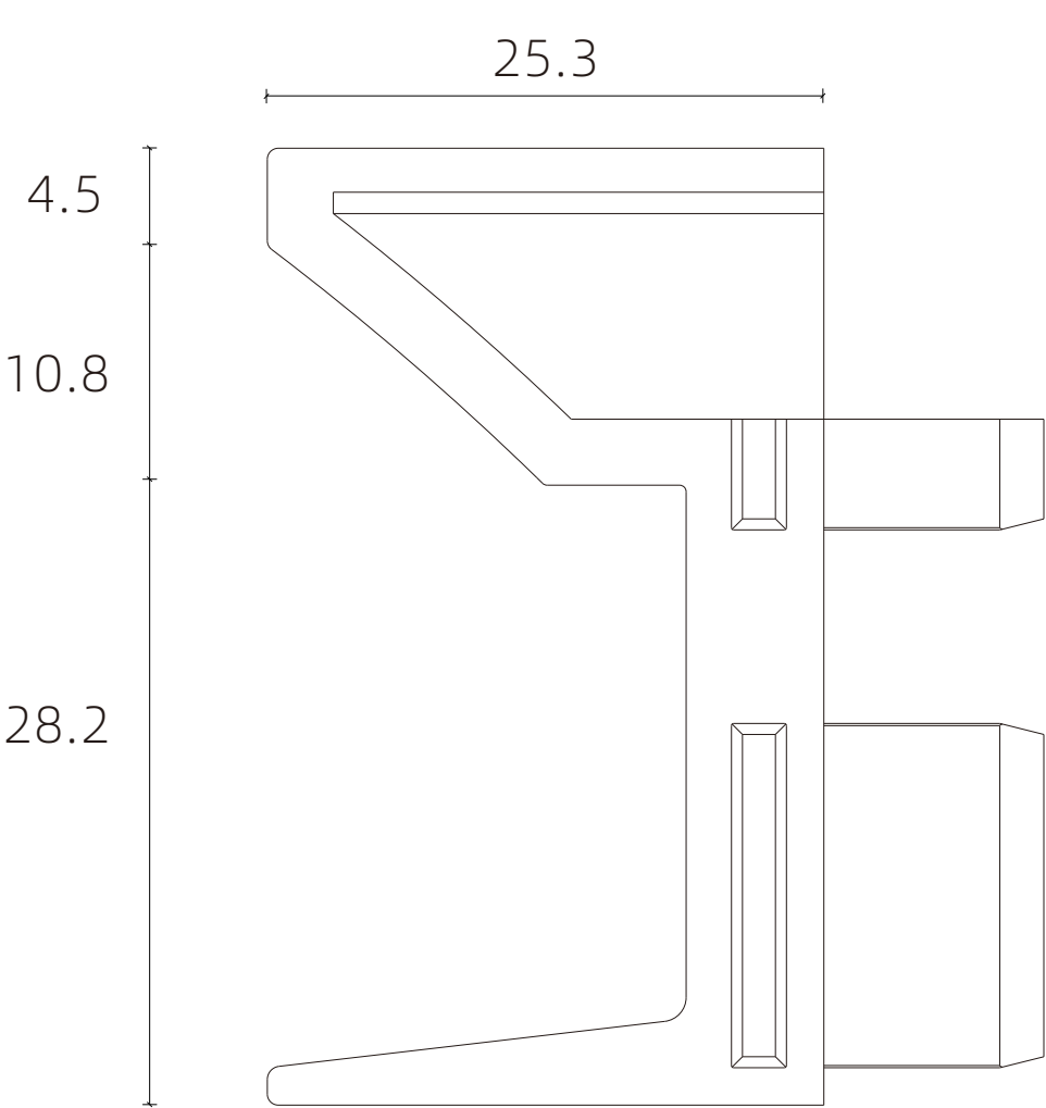
D4325锌转角连接件截面
