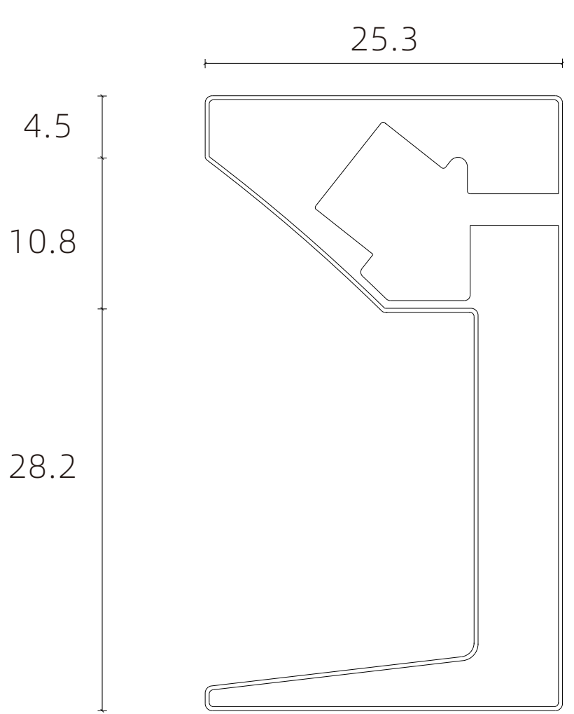
D4325锌端盖
