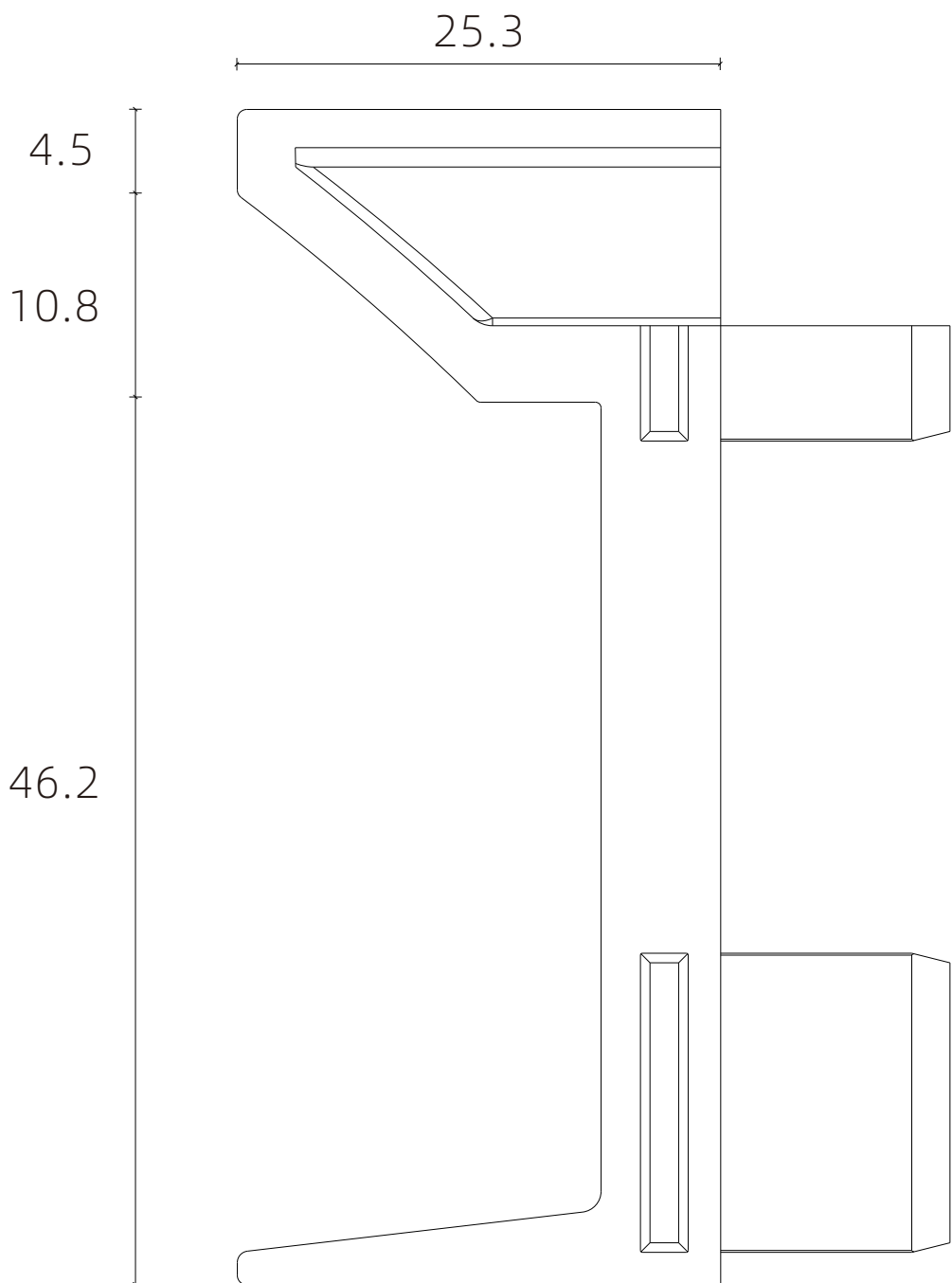
D62325锌转角连接件截面
