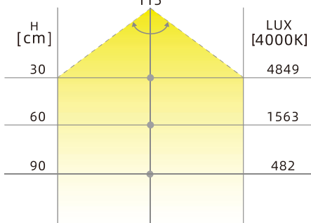
D25 照度值（勒克斯）
