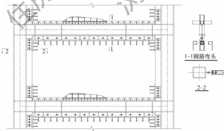
图 6.1.3 预制钢筋混凝土墙板与钢梁的连接
