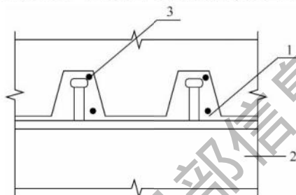
图 7.2.7 墙板底部与钢梁齿槽栓钉连接
