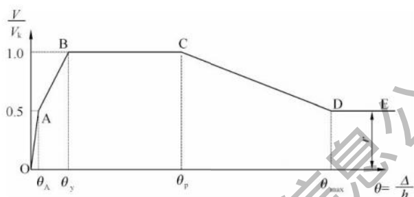
图 6.1.11 墙板侧向荷载-位移关系曲线
