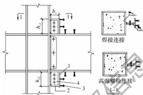
图 7.2.3 梁柱节点角部抗剪加强板
