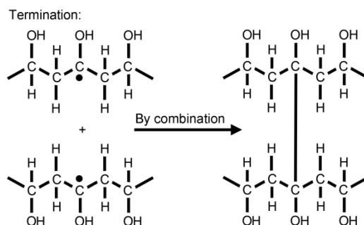
图5 辐射交联PVA水凝胶的主要反应机理
