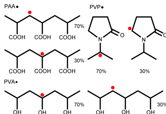
图4 PVA、PAA、PVP形成的初级自由基及比例
