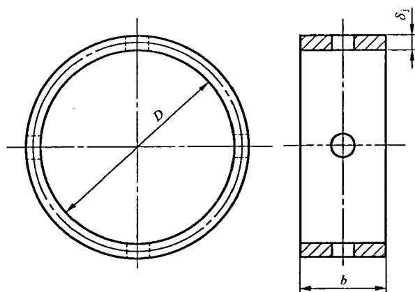
图 C.7 圆形万向环
