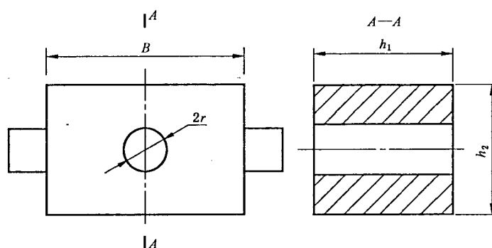
图 C.6 十字销轴
