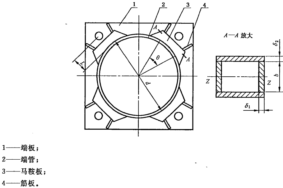
图 C.10 有筋板的端板
