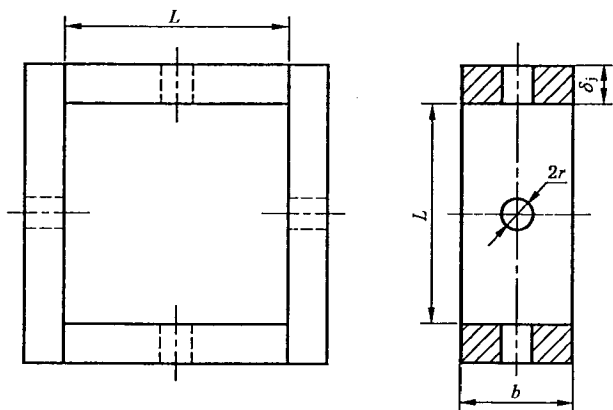
图 C.8 方形万向环
