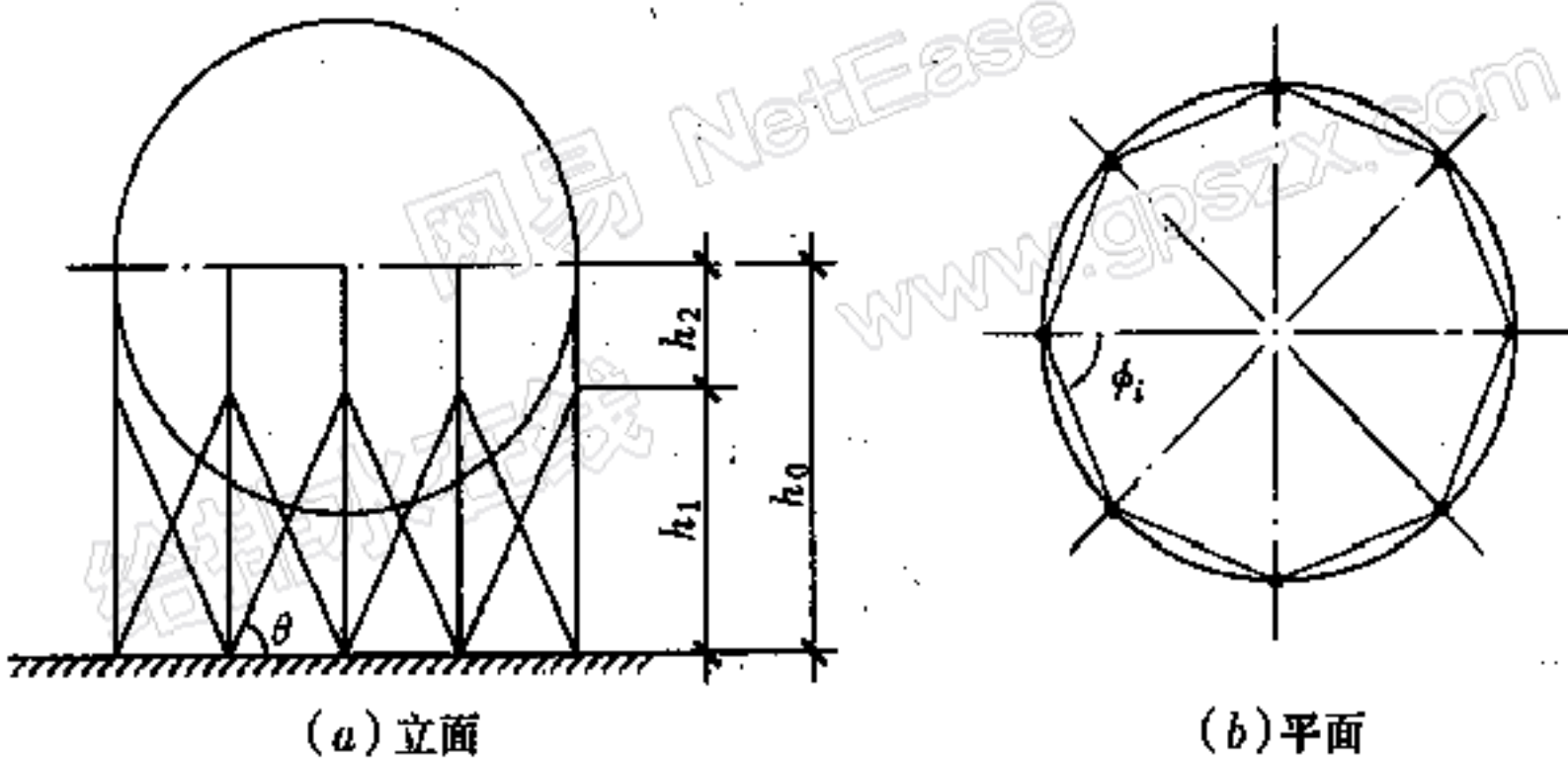
图 7.2.3 球罐简图
