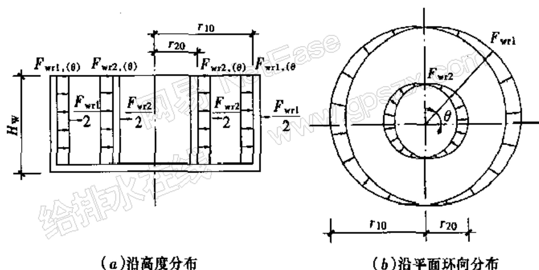
图 7.4.4 环形水槽动水压力
