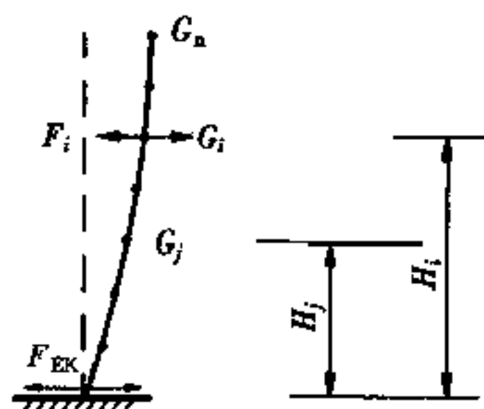
图 5.2.1 水平地震作用计算简图
