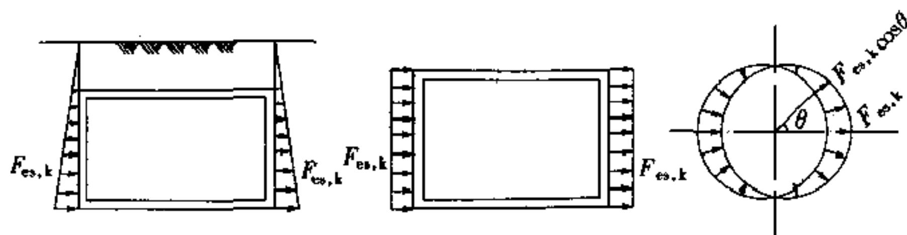
(a)沿高度分布 (b)矩形水池沿平面分布 (c)圆形水池沿平面分布
