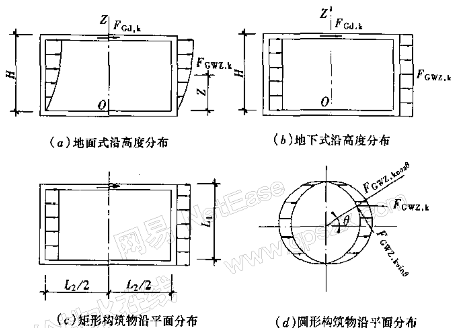
图 6.2.1 自重惯性力分布图
