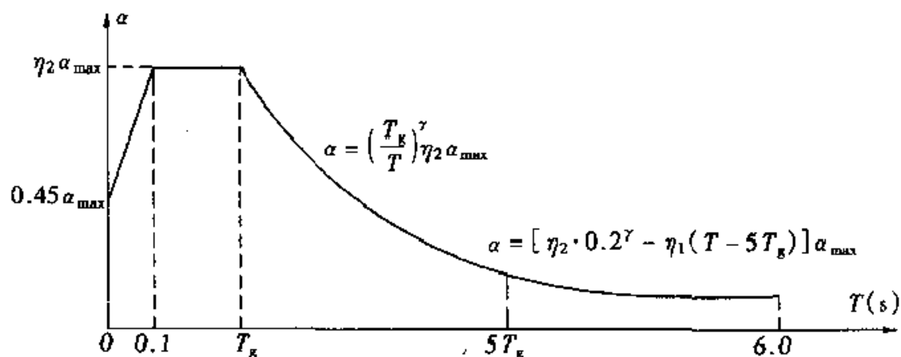
图 5.1.5 地震影响系数曲线
