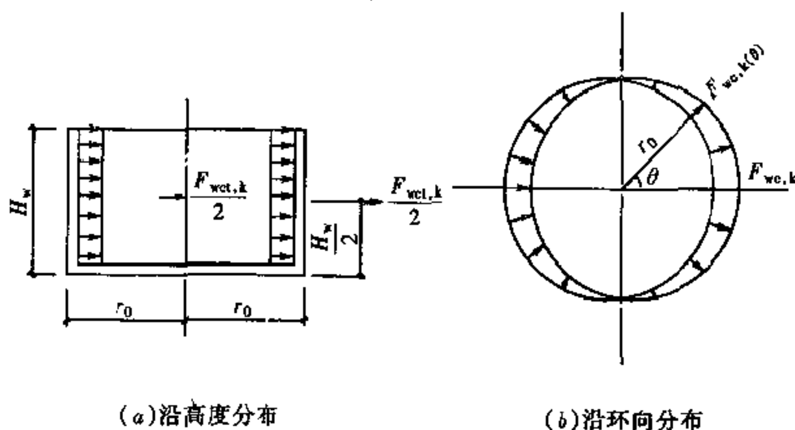
图 6.2.2 圆形水池动水压力
