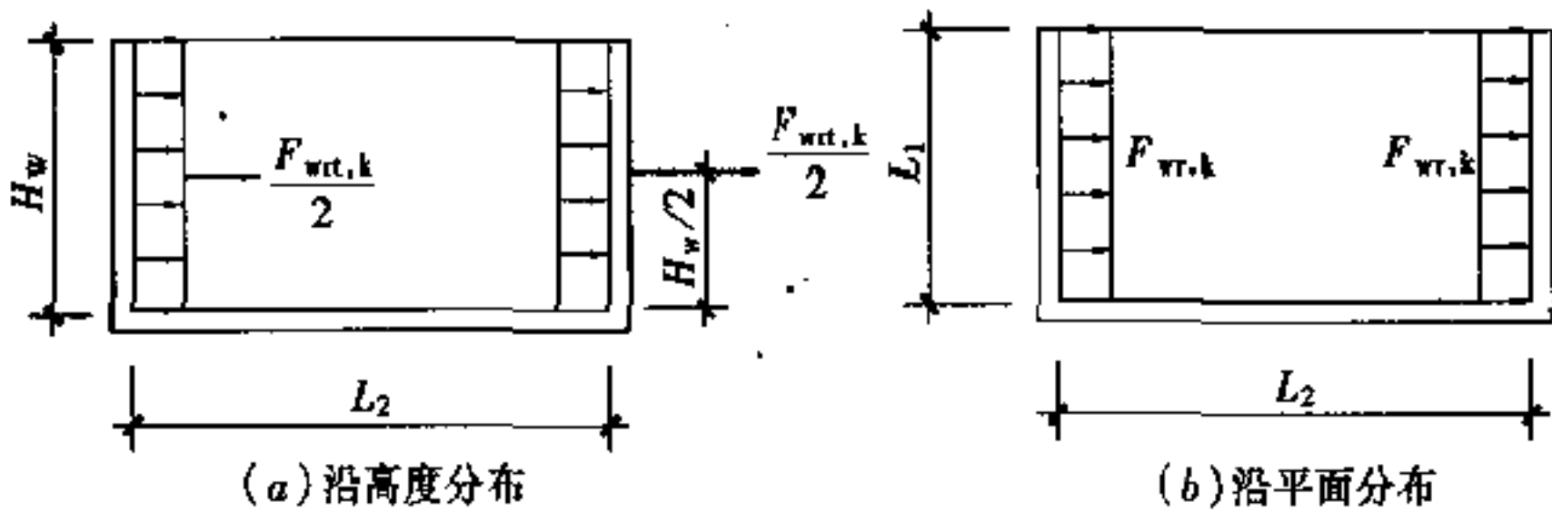
图 6.2.3 矩形水池动水压力
